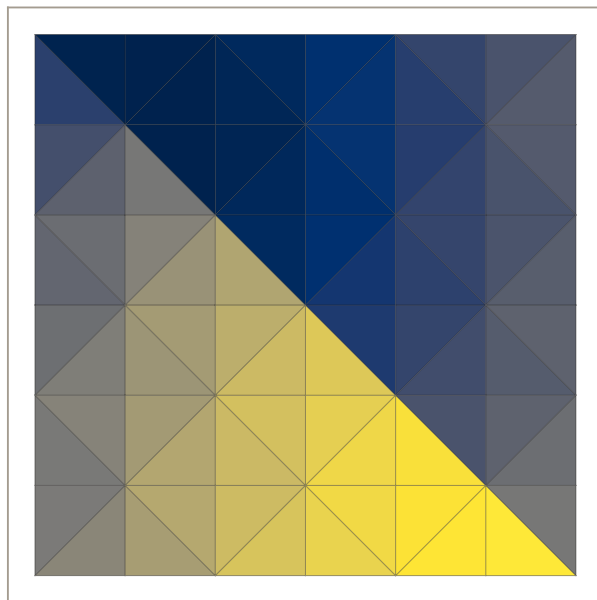
(d) piecewise-smooth field
