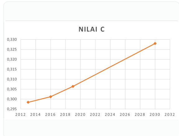
Tren Nilai Koefisien Limpasan (C)
