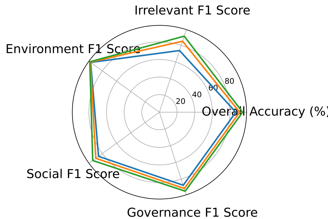
BERT-base-multilingual
