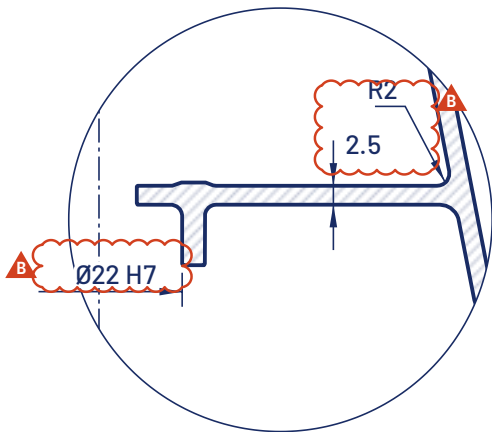
FIG. 2 DETAIL A · 1:1
