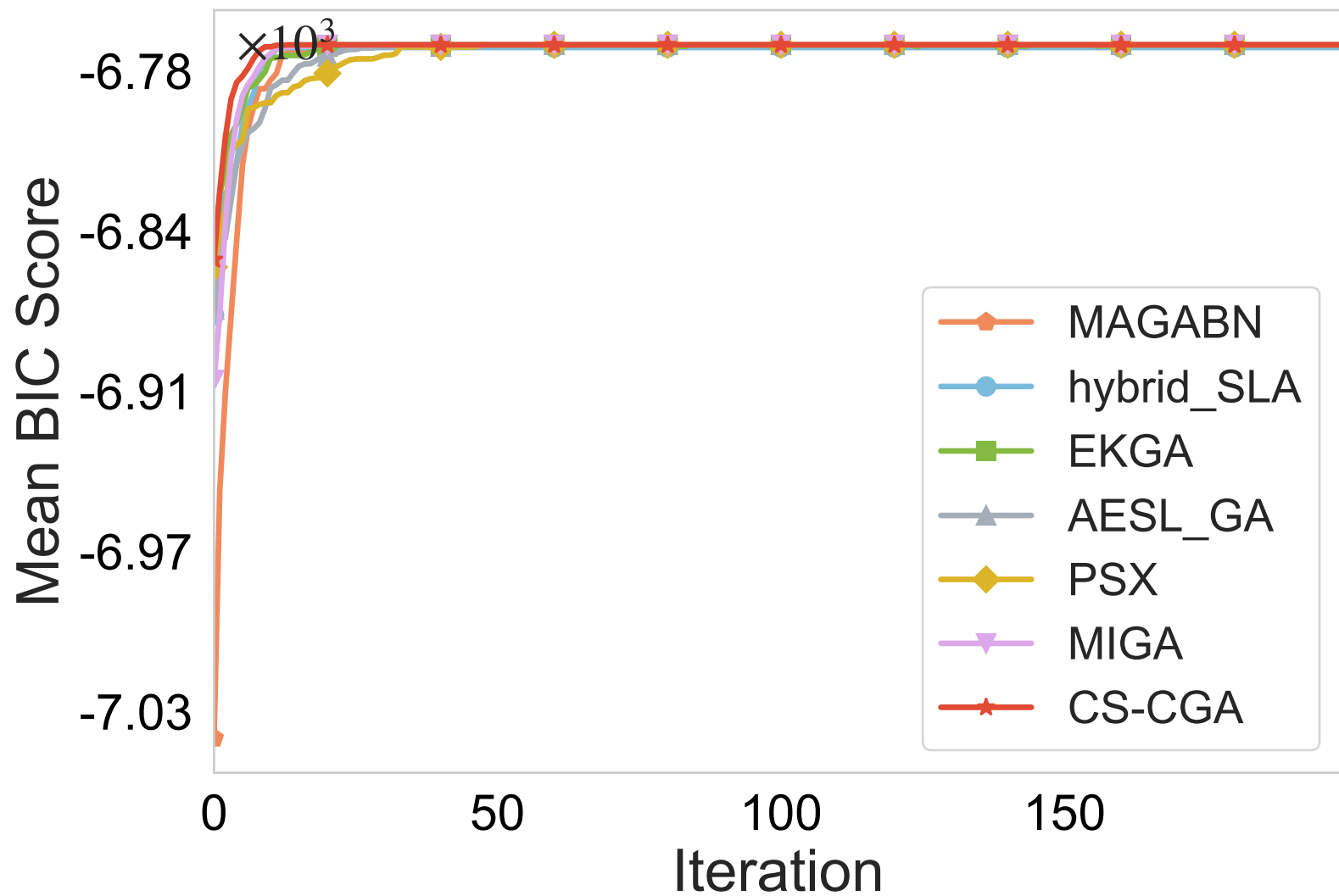
BIC Convergence - AS-3000
