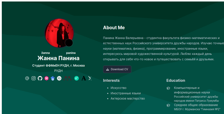
Рис. 7: Проверка изменений
