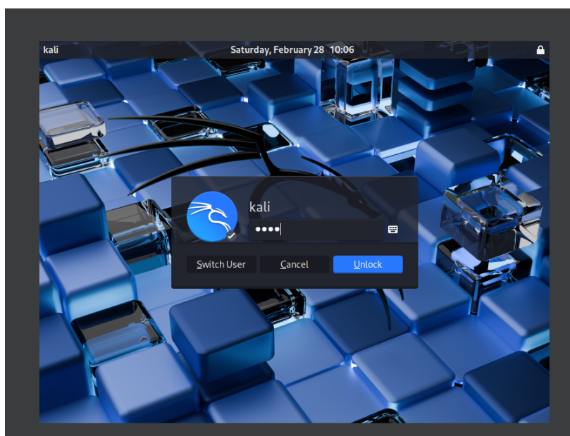
Рисунок 4.7: Вход
