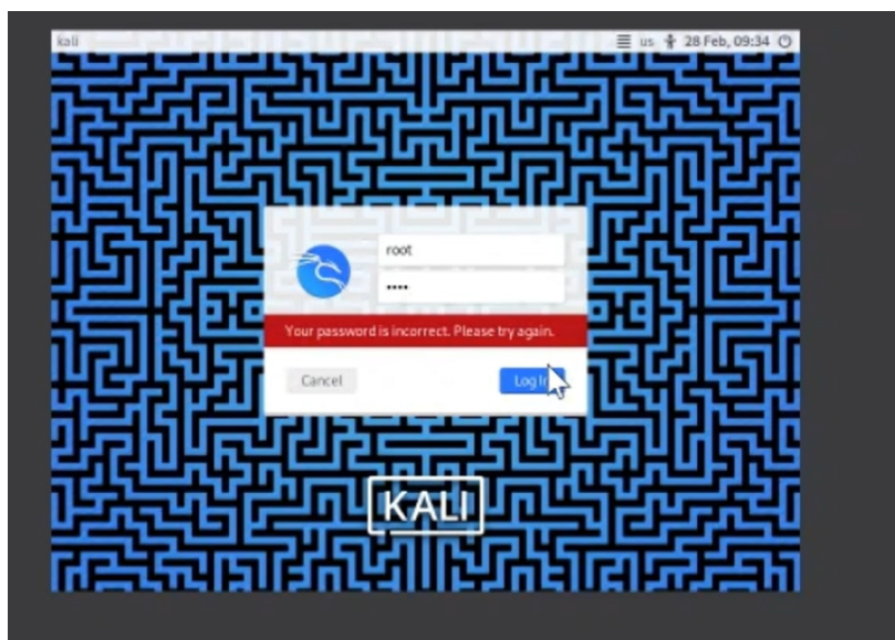
Рисунок 4.6: Вход
