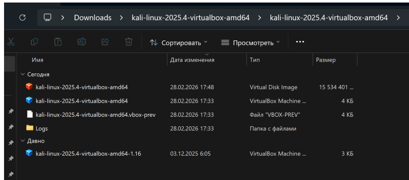
Рисунок 4.4: Распакованные файлы
