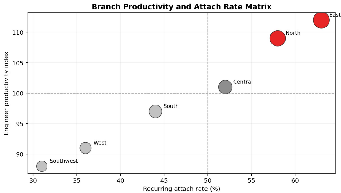
图 2 分公司生产率与服务渗透率矩阵
