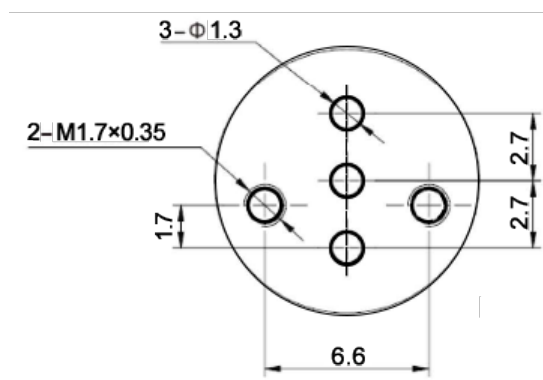
孔位安装图
