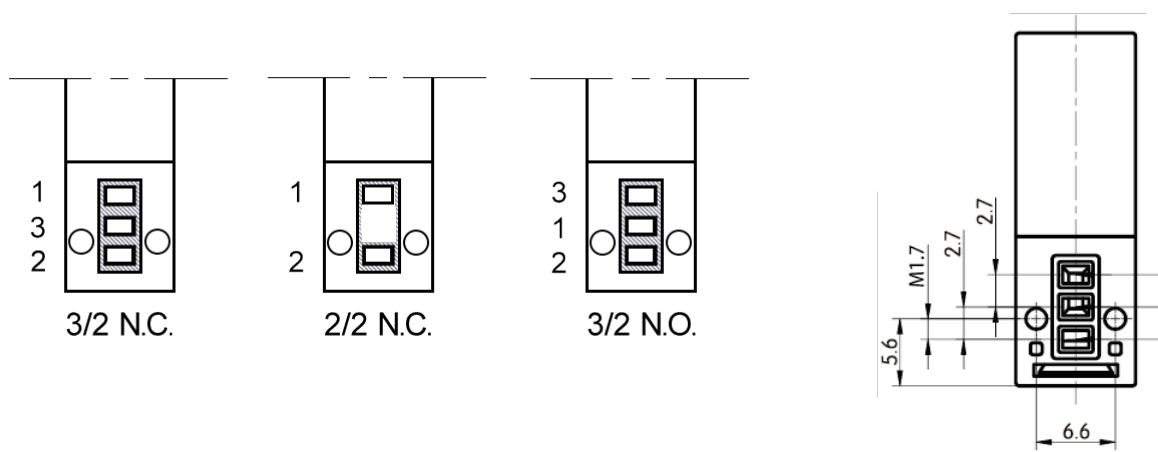
底部尺寸
