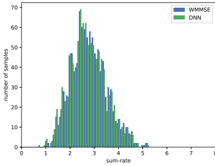
图 5: IC 信道 K = 10
