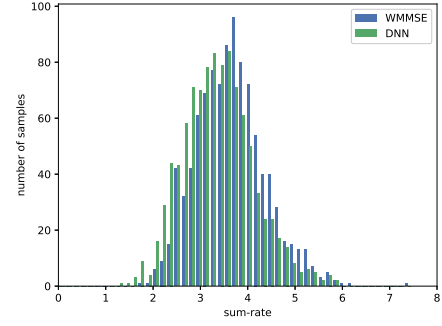
图 6: IC 信道 K = 20
