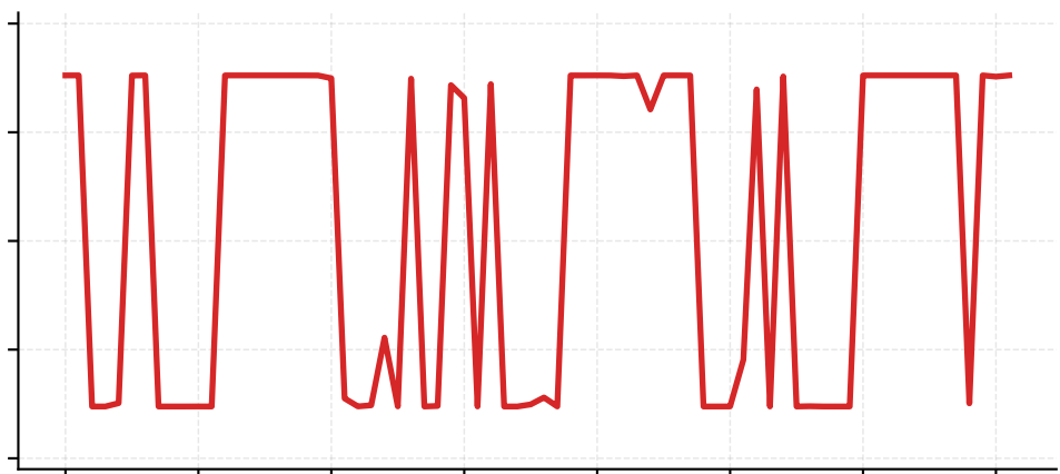
SAC
