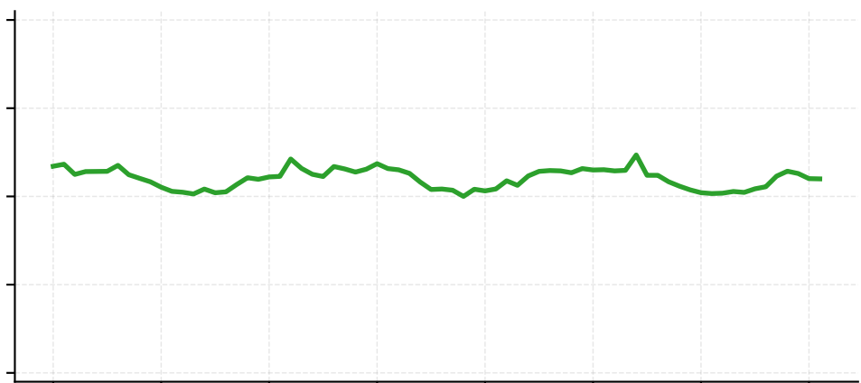
SAC
