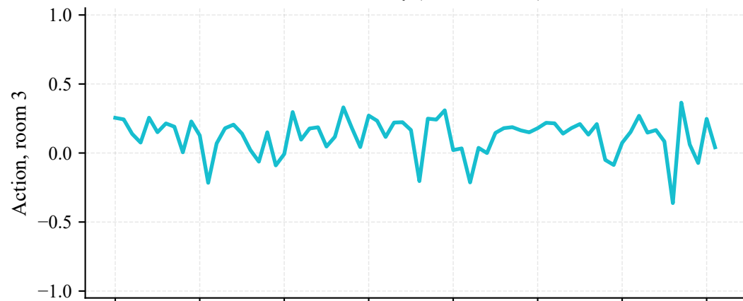
SAC+MPC
