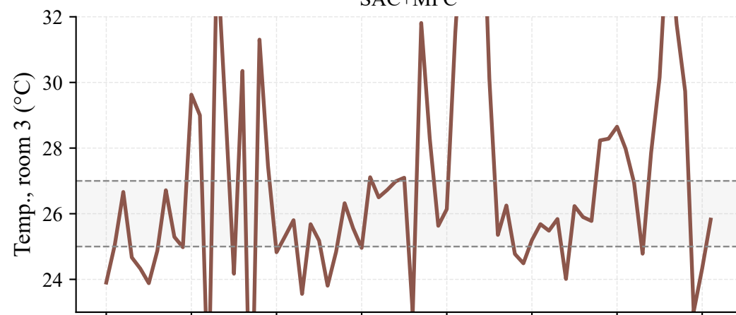
SAC+MPC
