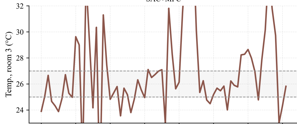
SAC+MPC
