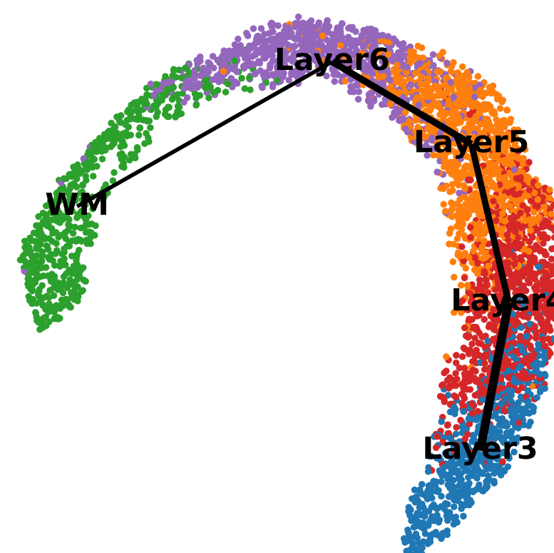
Spatial-MGCN
