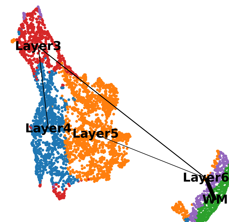
spaVAE
