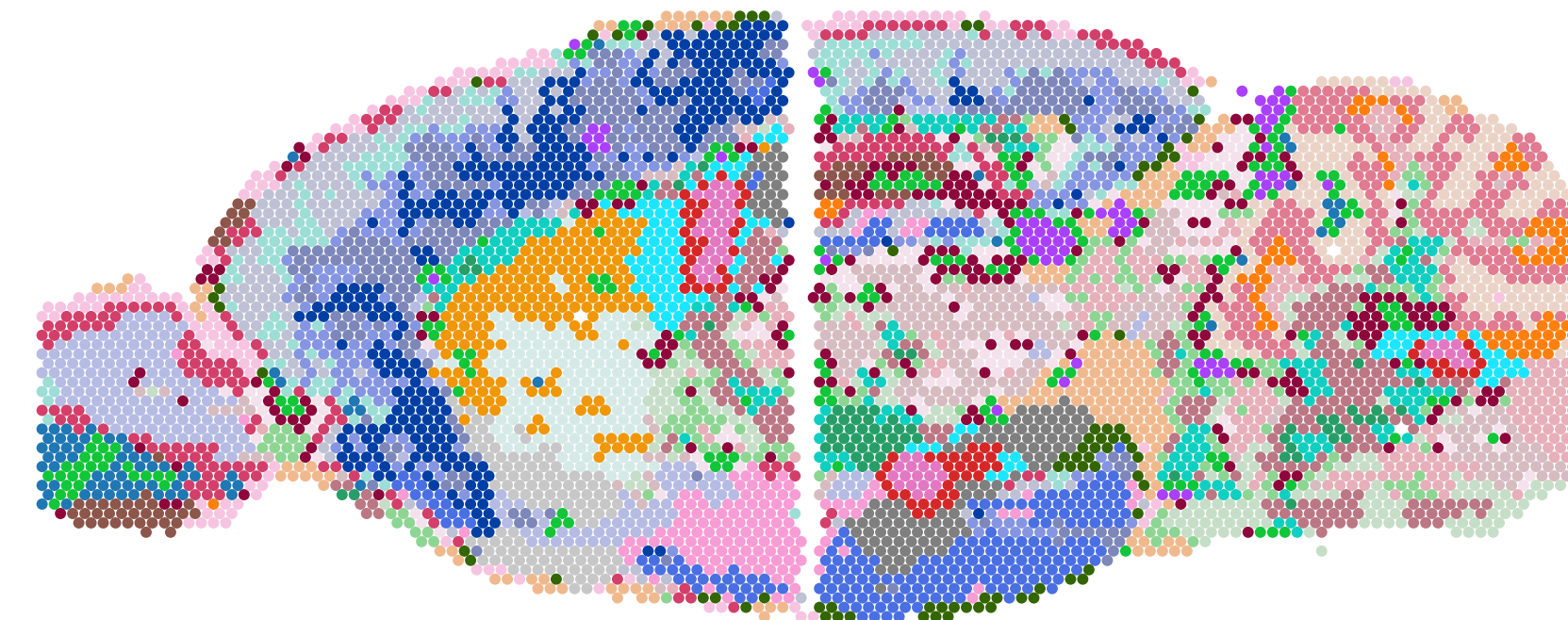
SpatialMGCN
