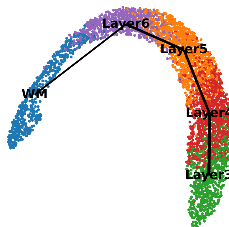
SpaGCN
