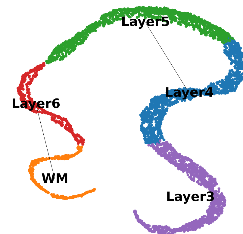
GatorTrio
