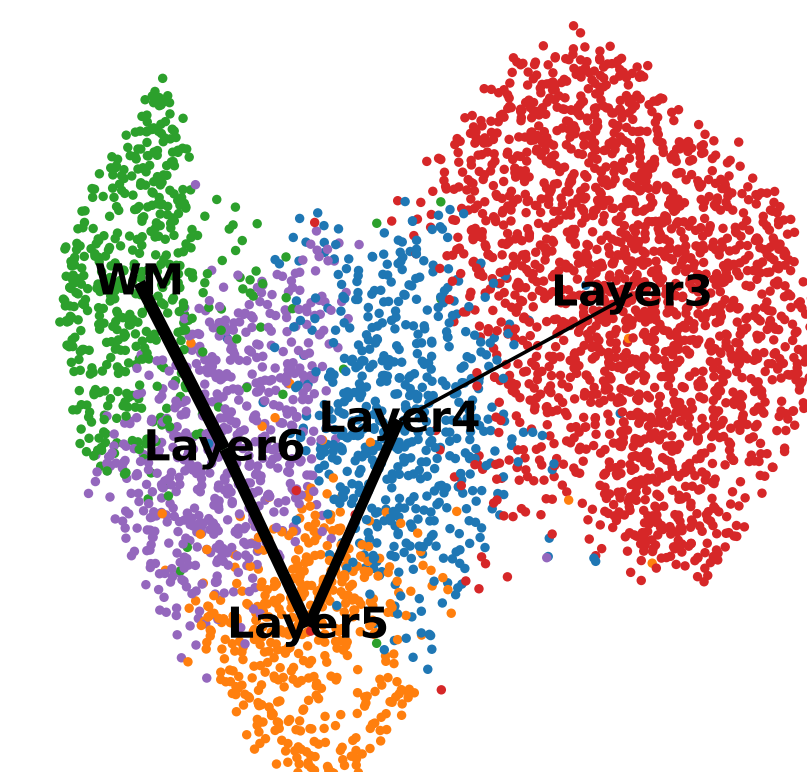
GatorTrio
