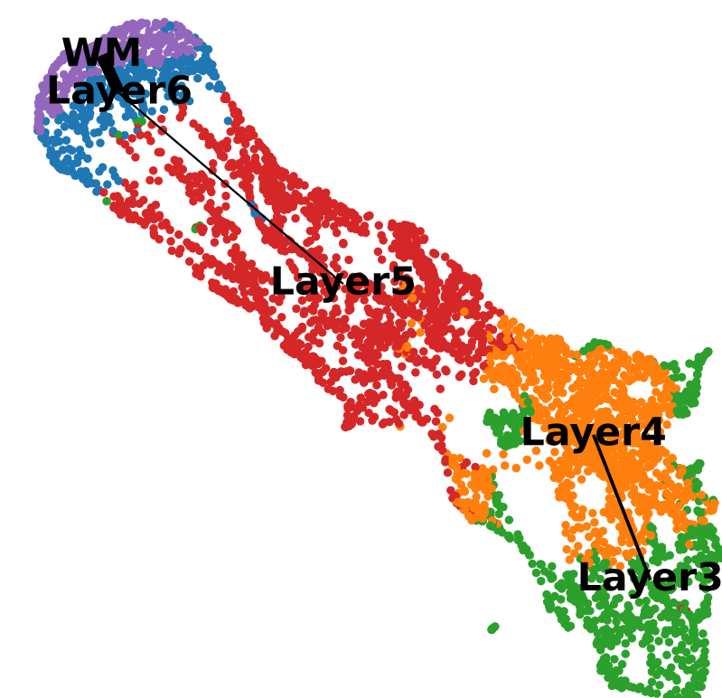
NichePCA
