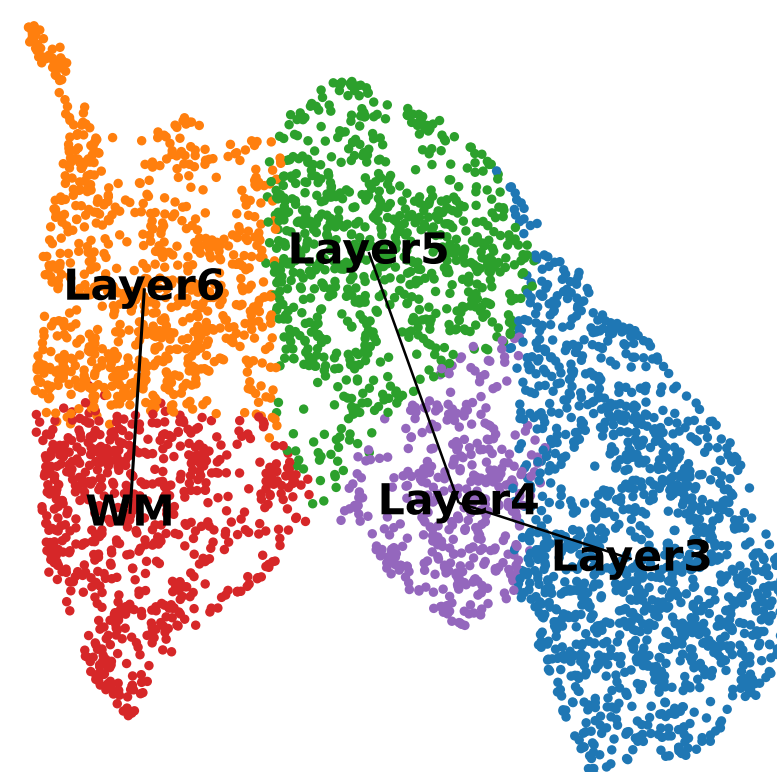
Spatial-MGCN
