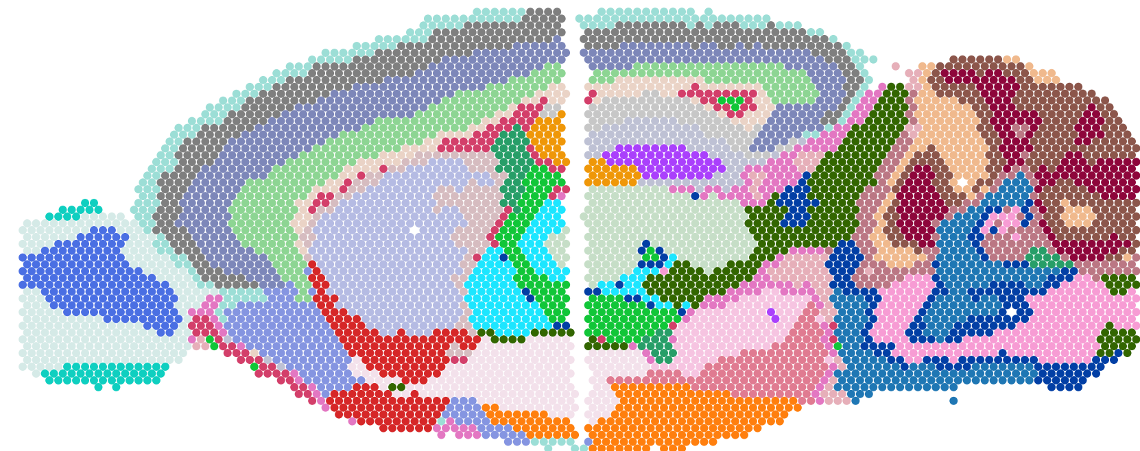
spaVAE
