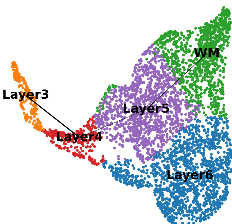
spaVAE
