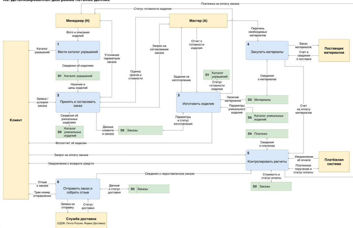
А0. Детализированная диаграмма потоков данных
