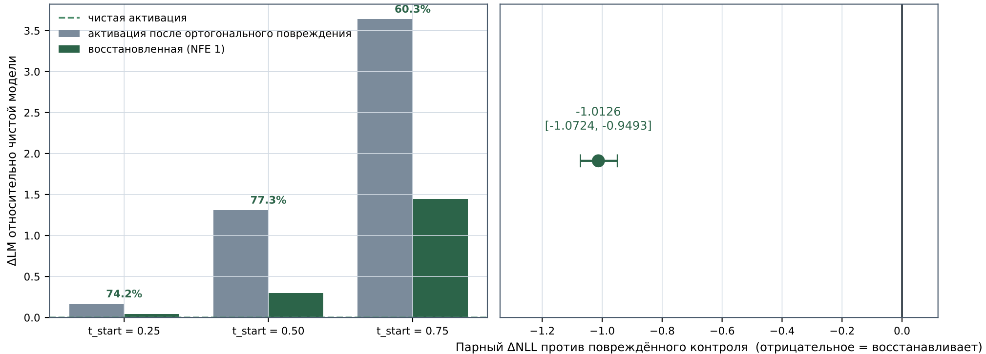
A. Восстановление своей же задачи (подпись — доля восстановленного) В. Критерий T1 выполнен ( t = 0.50 , NFE 1)
