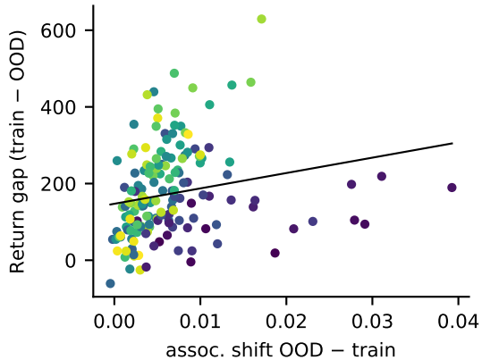
Color shift ( r = 0.20 , n = 162 )
