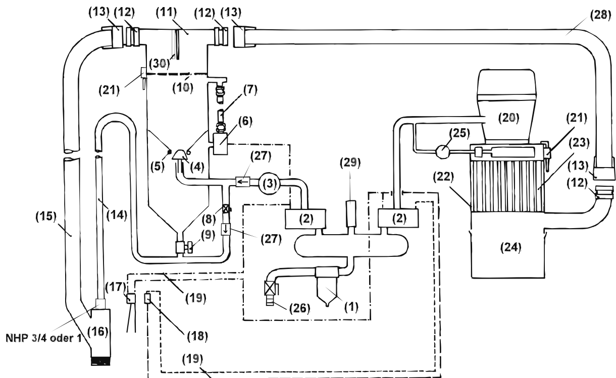
Заменяемые части HS 200P-1
