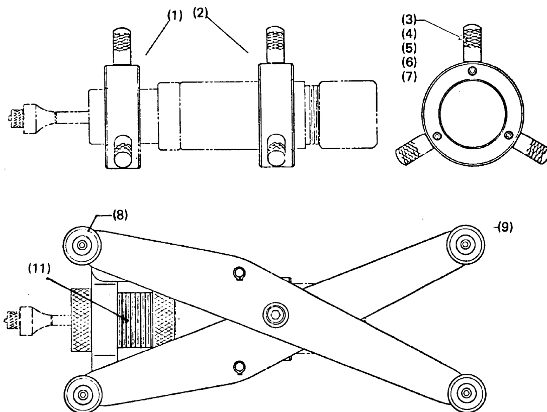
Центрующее устройство и вагонетка для Hollo Blast
