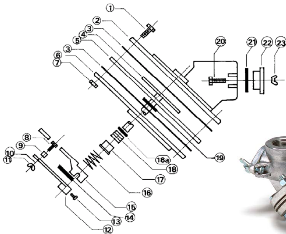
Дозирующий клапан FSV
