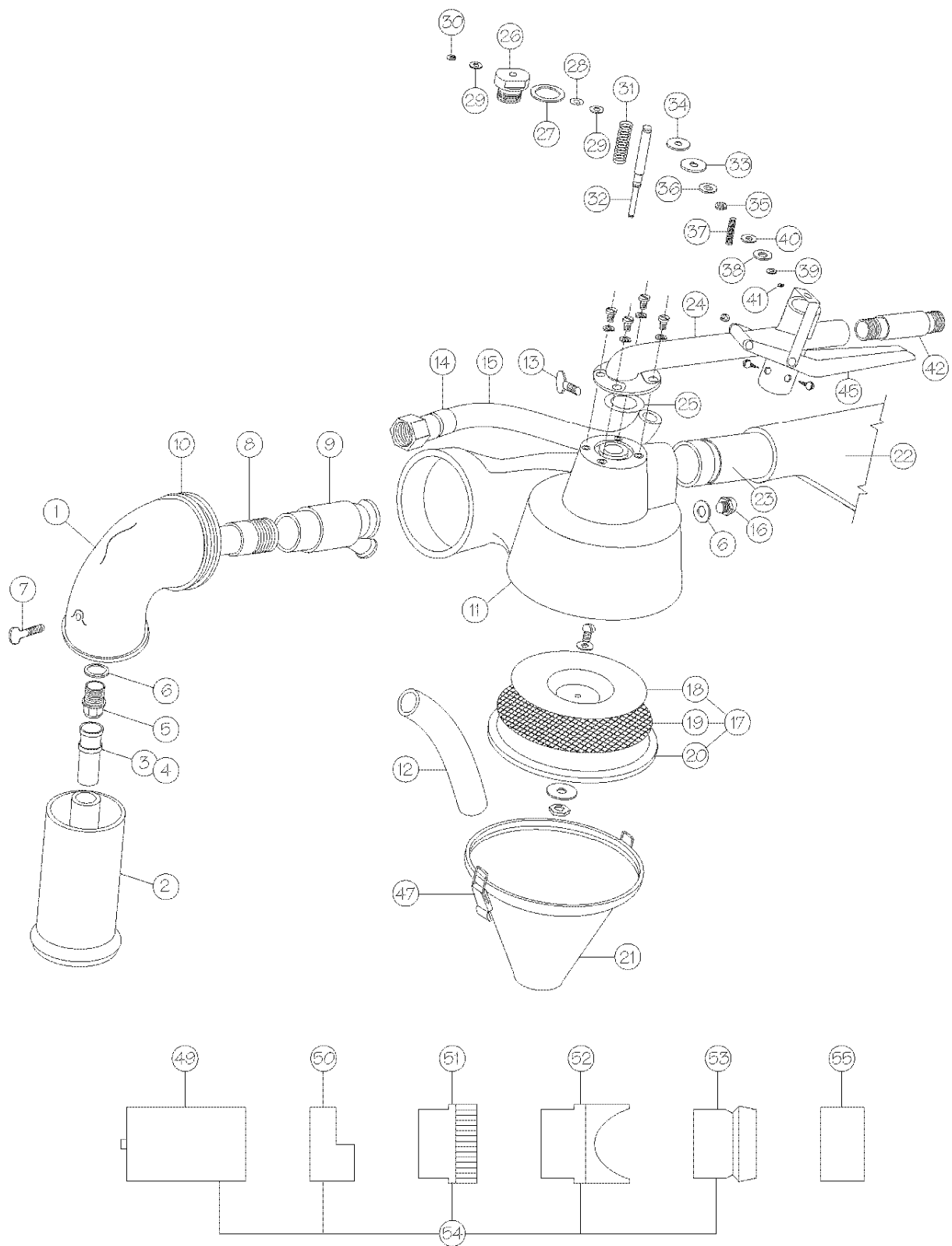
Заменяемые части Educat-O-Matic
