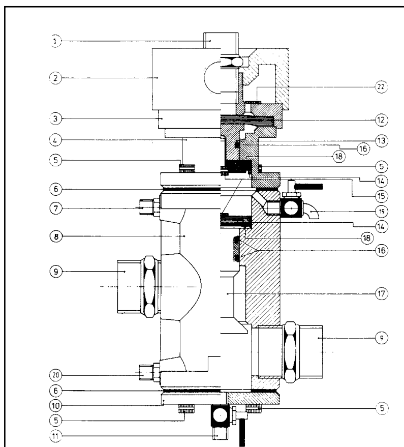
Клапан дистанционного управления RMS-100
