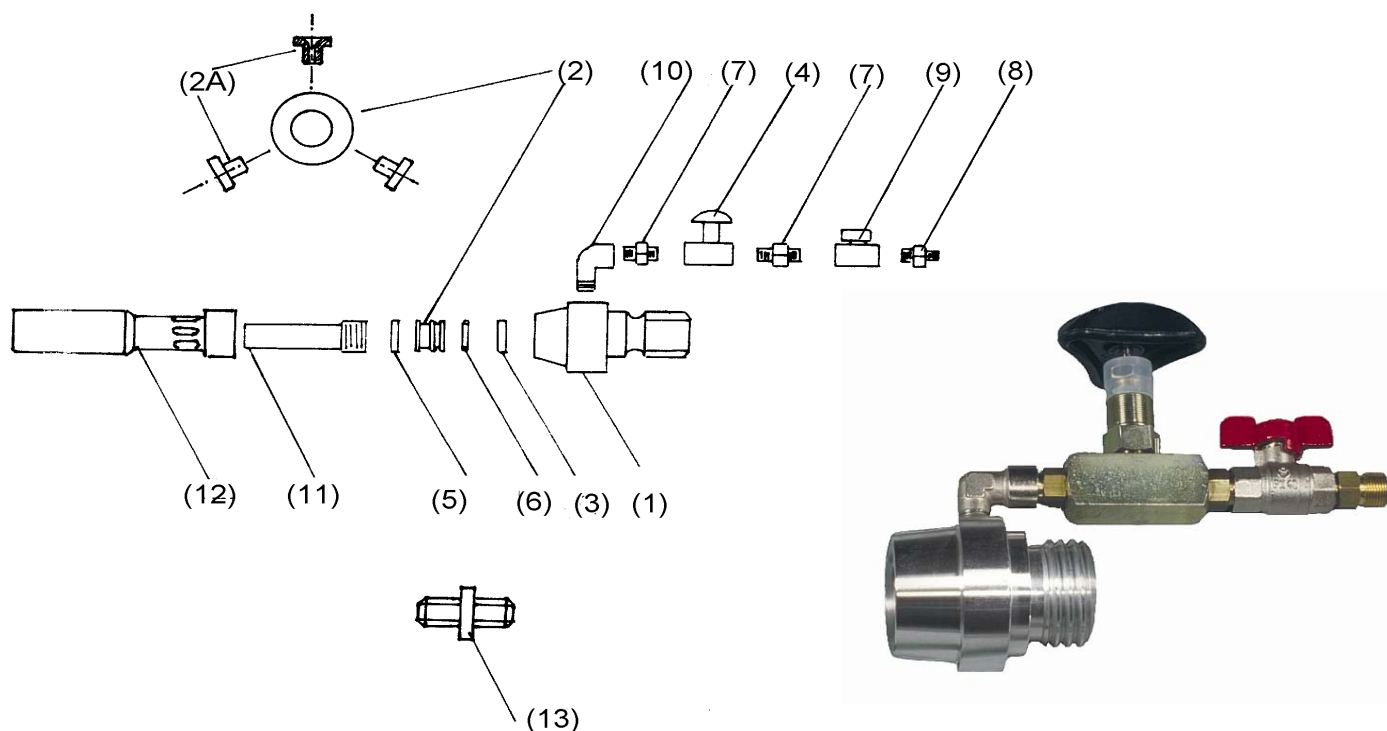
Головка для влажной очистки KB 52-1
