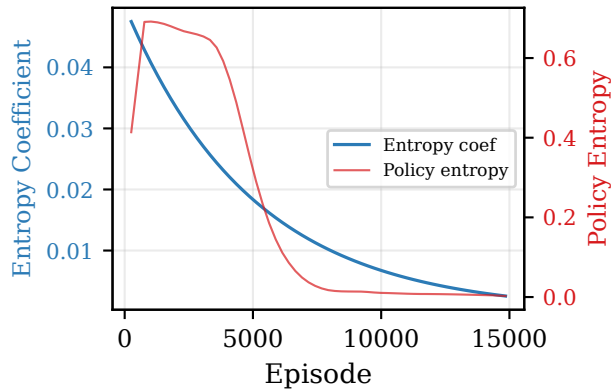
(d) Exploration Decay
