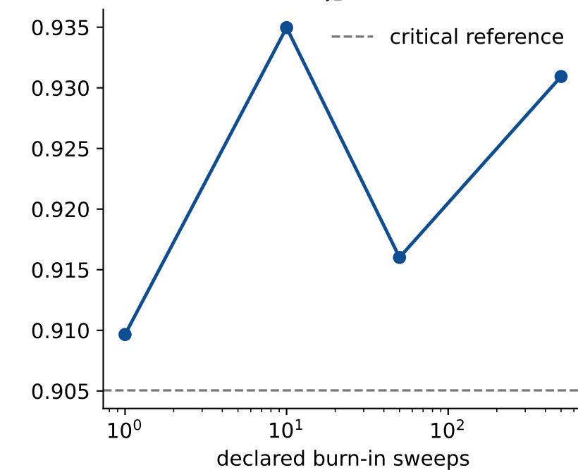
\xi_2/L
