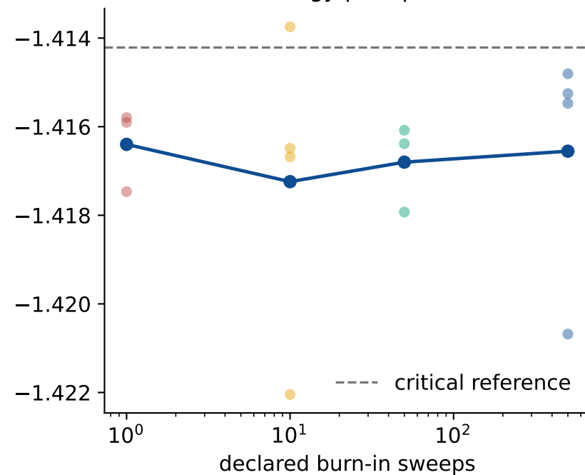
Energy per spin
