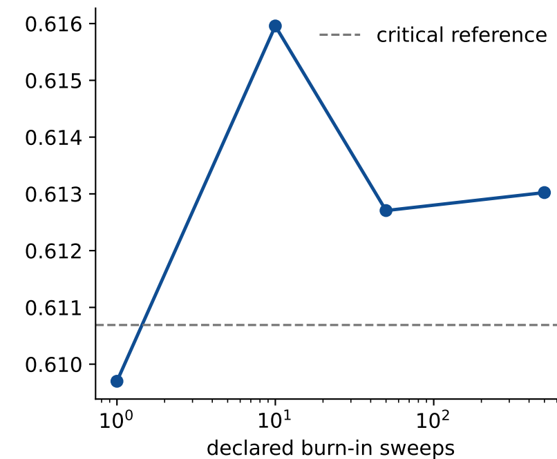
Binder U_4
