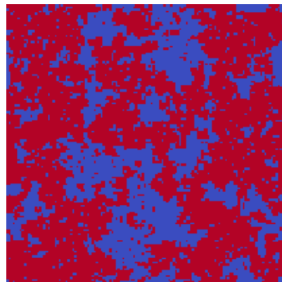
L=128 MC m=+0.29
