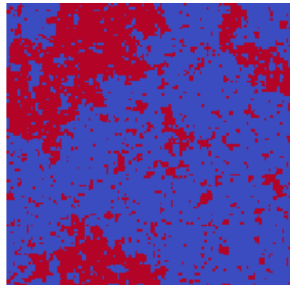
L=128 MC m=-0.67
