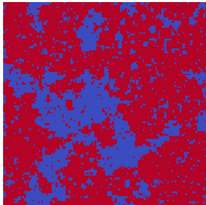
L=128 MC m=+0.01
