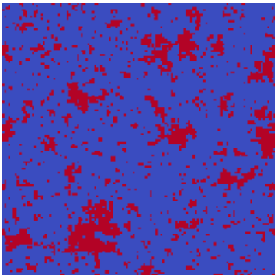
L=128 MC m=-0.69
