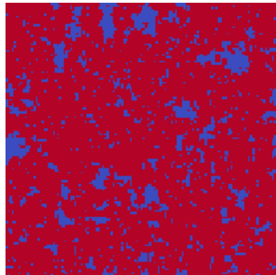
L=128 MC m=-0.65
