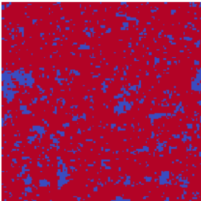
L=128 MC m=+0.56
