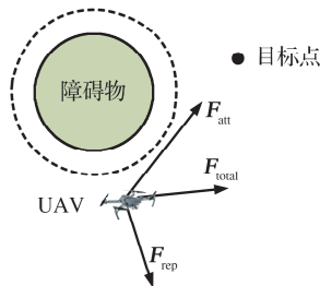
图 3 人工势场受力模型
