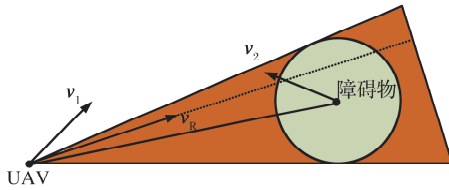
图 4 速度障碍法冲突解脱示意图
