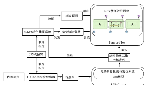
图 2.1 系统整体框架
