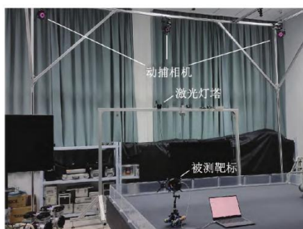
图 4 位姿测量精度测试
