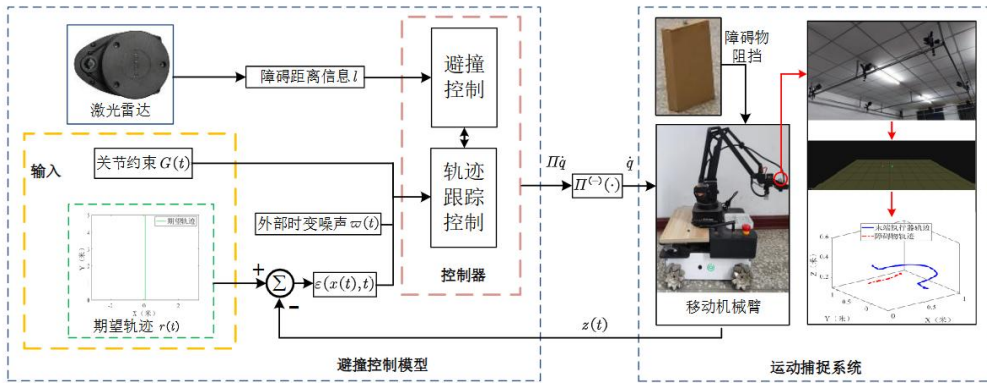
图 4.6 避撞控制模型 (4-10) 平台实验验证框图
