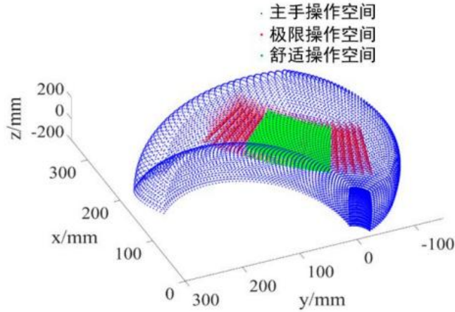
图 5.3 主操作手工作空间与人手操作空间
