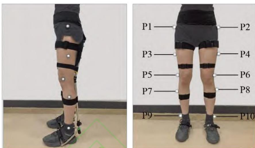
图 2 Mark 点粘贴示意图
