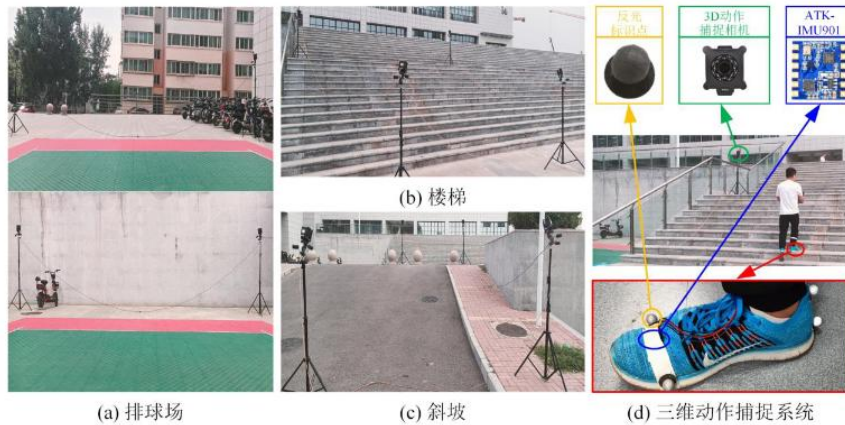
图 3-10 利用光学三维运动捕捉系统获取试验的真实参考
