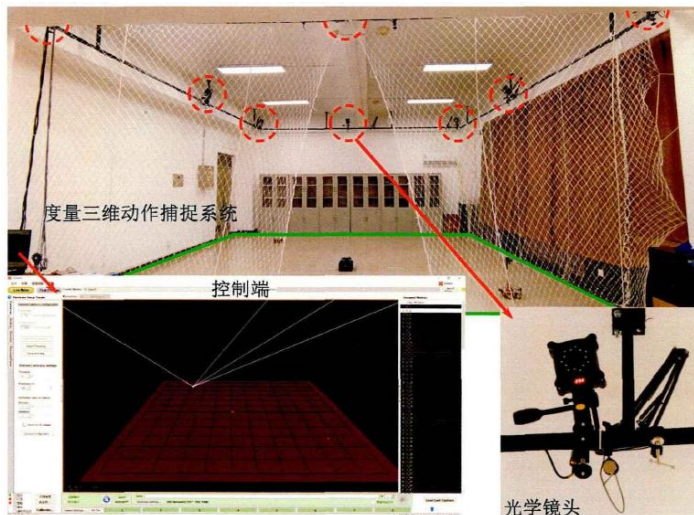
图 6-1 度量光学三维动作捕捉系统
