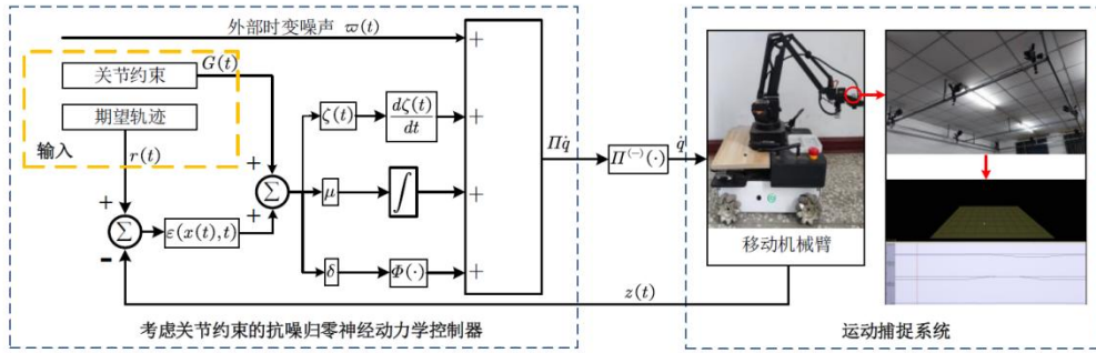
图 3.14 NSZNN-JAC 模型 (3-15) 平台实验验证框图
