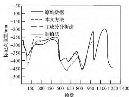
图5 连续丢失 800 帧的数据修复结果
