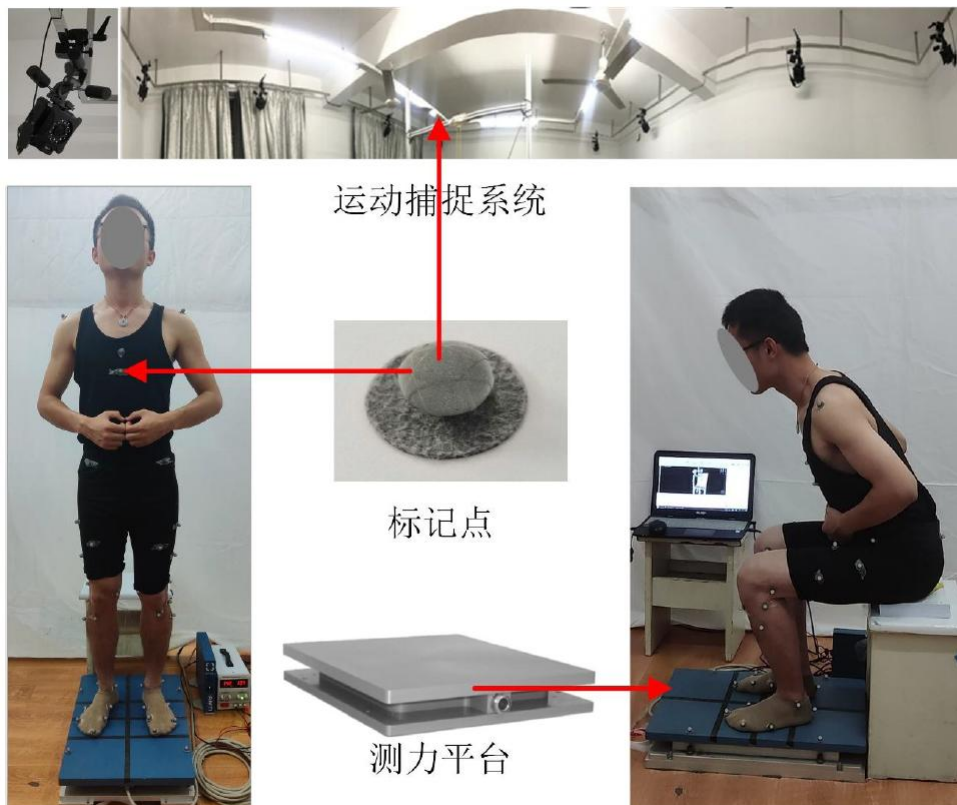
图 3-5 人体起立实验平台
