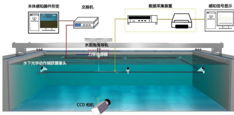
图 4.5 动作捕捉区域 Figure 4.5 Motion capture area
