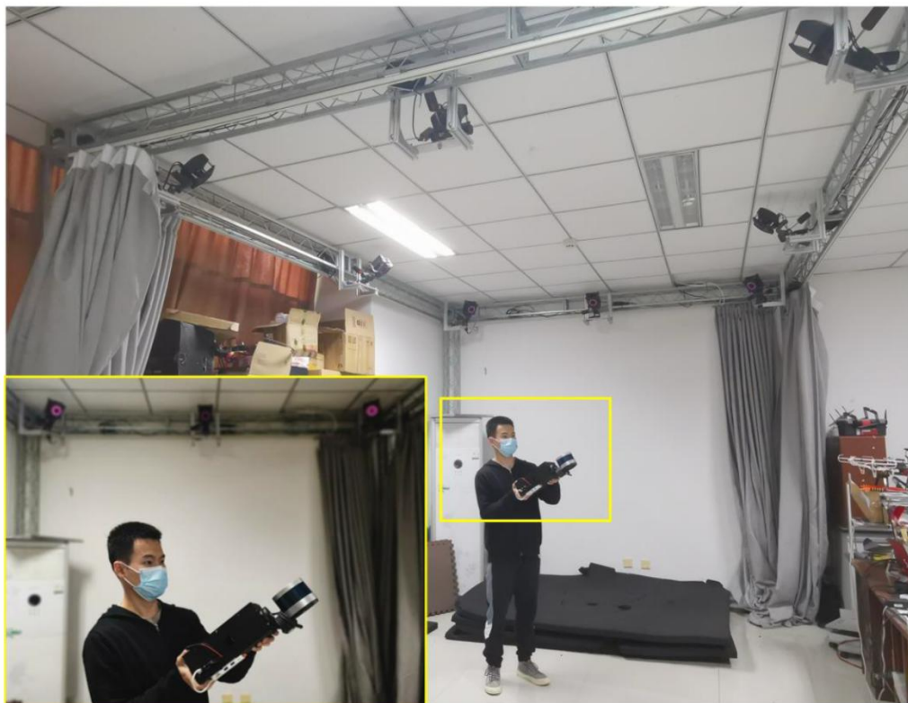
图 4-3 Nokov 运动捕捉系统实验室
