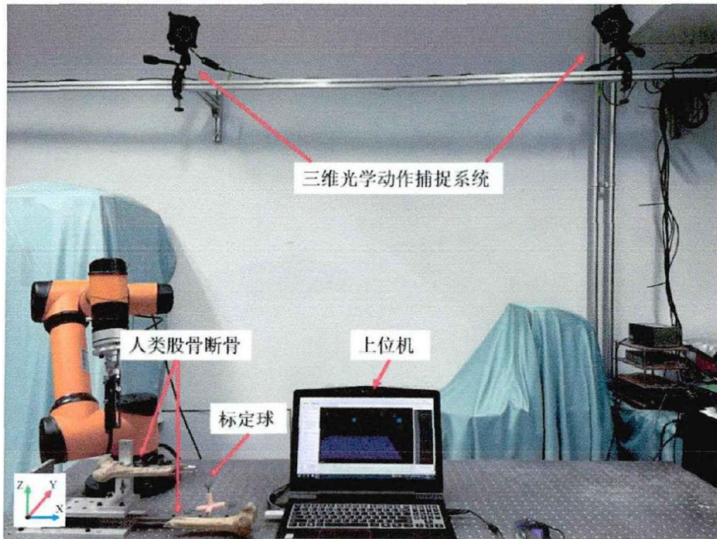
图 3-1 路径采集平台示意图
