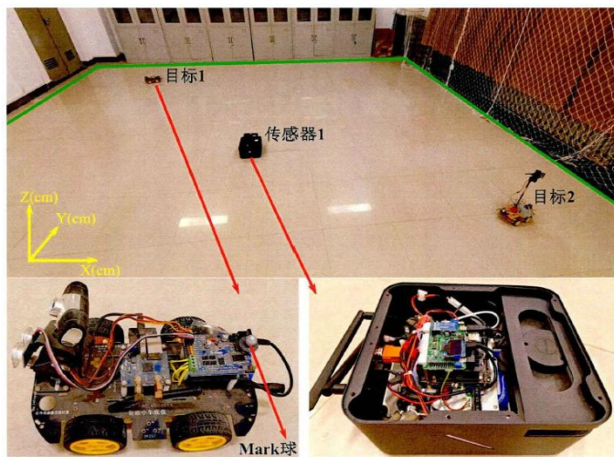
图 6-2 初始场景，全向麦轮小车(右)与智能小车(左)
