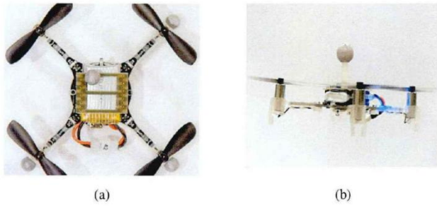
图 2-2 四旋翼无人机 Crazyfly Fig.2-2 Quadrotor: Crazyfly
