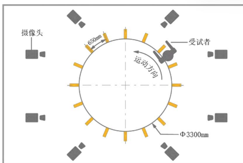
图 3 动捕场景示意图
