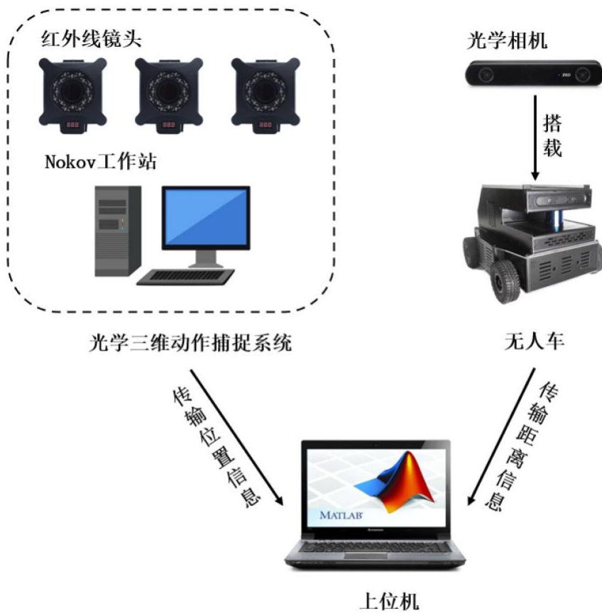
图 5-1 半实物验证平台系统框图及整体搭建示意图
