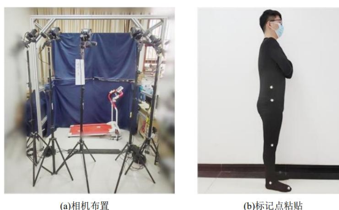
图2.4 Nokov 三维动作捕捉系统实验环境
