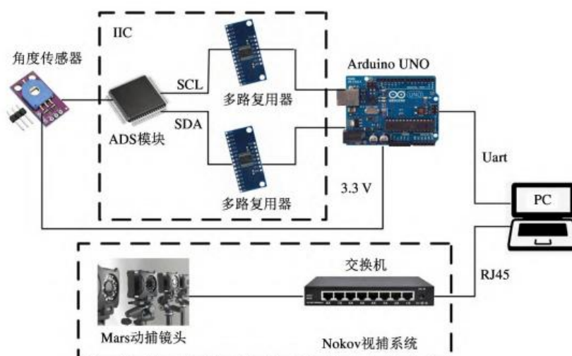
图7 硬件连接图
