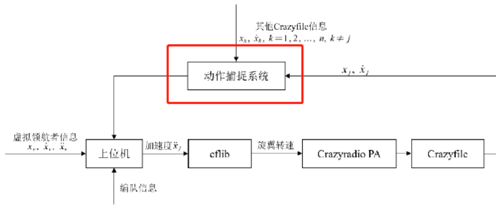
图 4-3 实验平台架构
