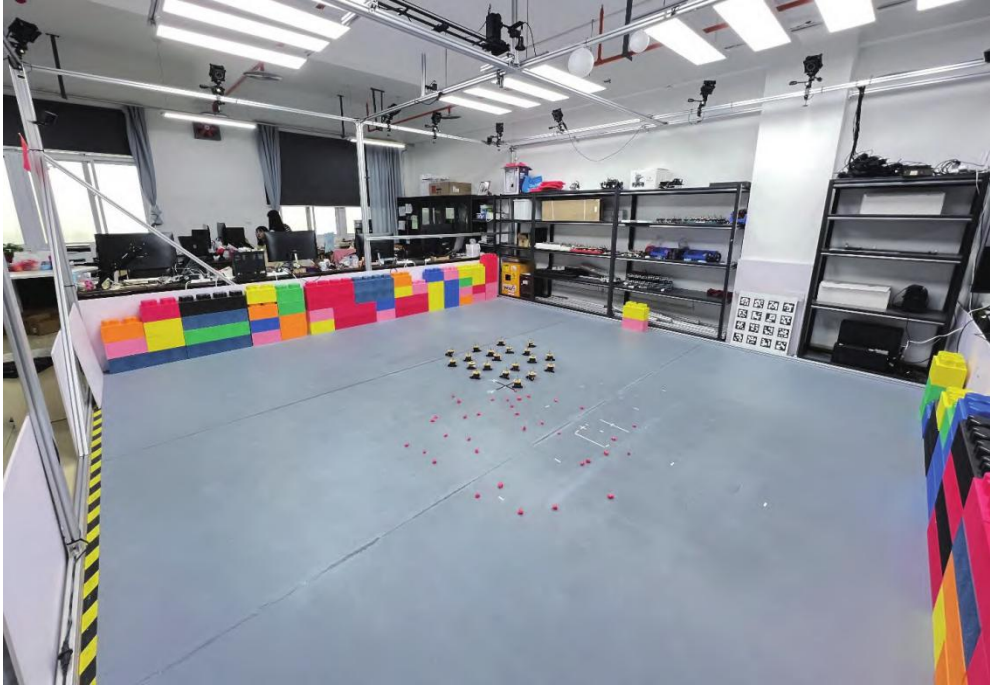
图 8 集群机器人与集群实验平台
