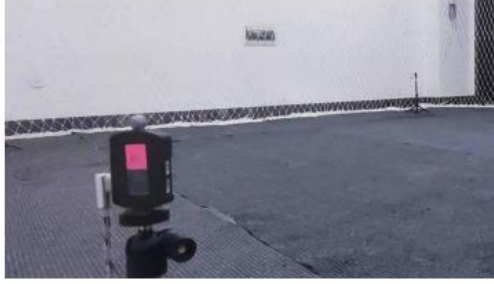
图 4-8 双领航者 UWB 基站实物图
