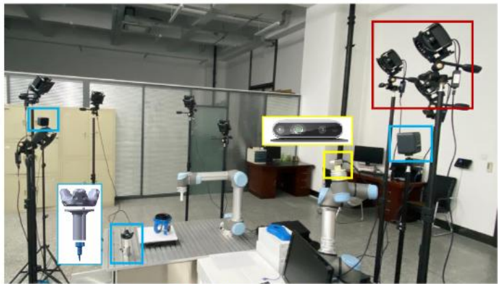
图 5-8 结合动作捕捉系统的平台搭建
