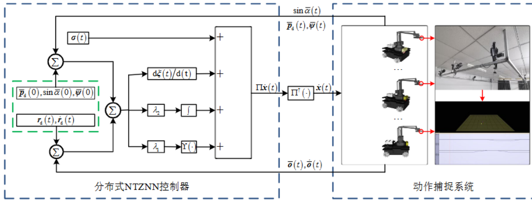
图 3.2 多全向移动机械臂协同运动控制流程图
