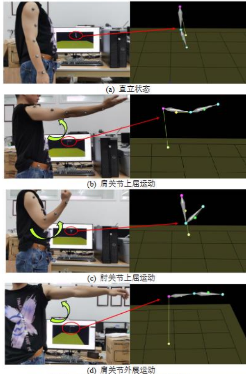
图 3-2 上肢康复运动实验姿态及刚体模型
