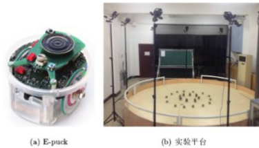
图 4.11 E-puck 机器人以及实验平台
