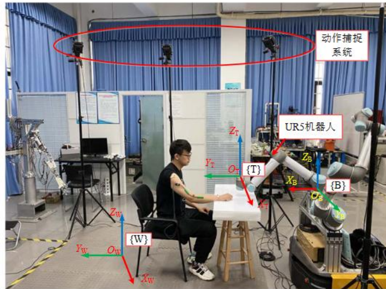
图 2-1 人机共存系统
