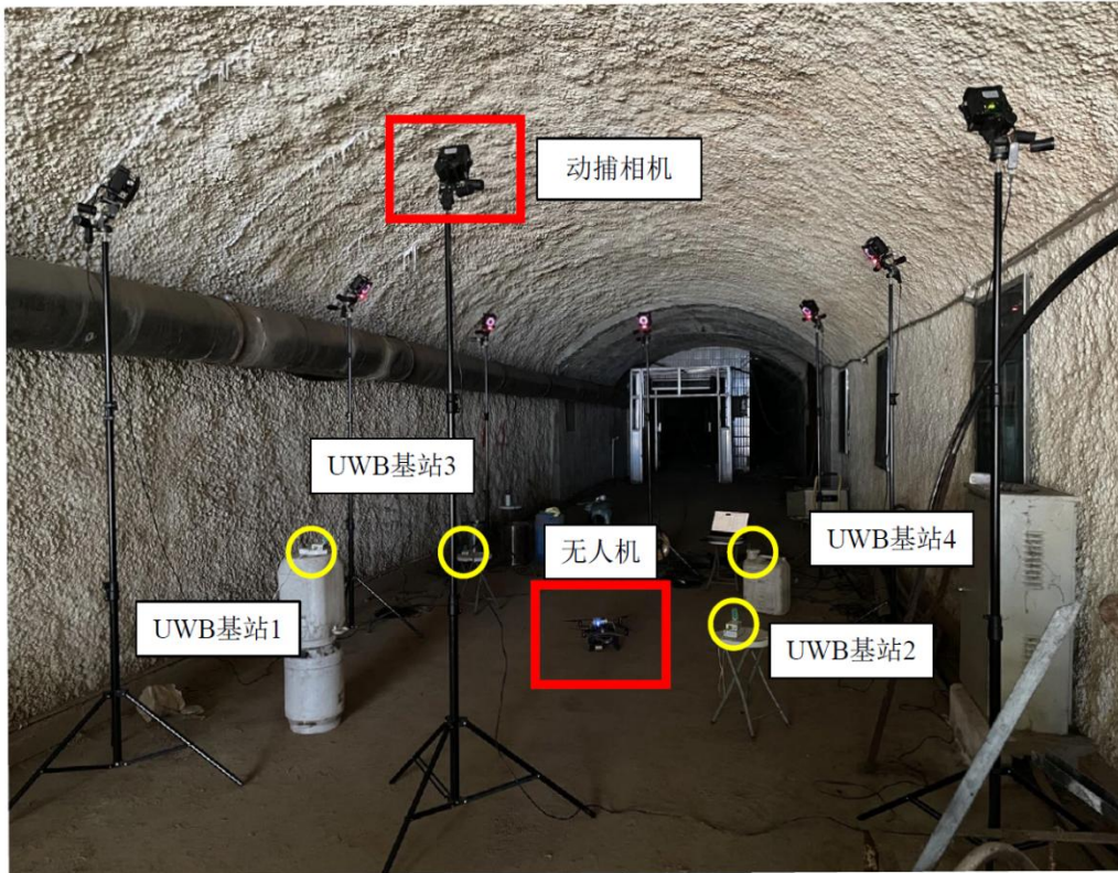
图 4-9 实验场景及设备部署
