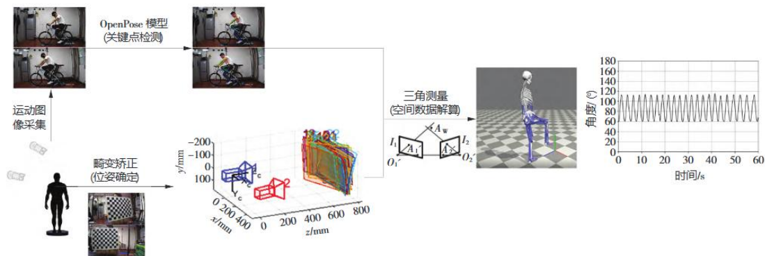
图 1 下肢运动检测系统设计整体流程图
