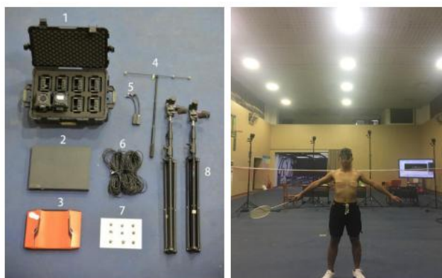
图 3-1 三维动作捕捉系统相关设备与受试者测试现场
