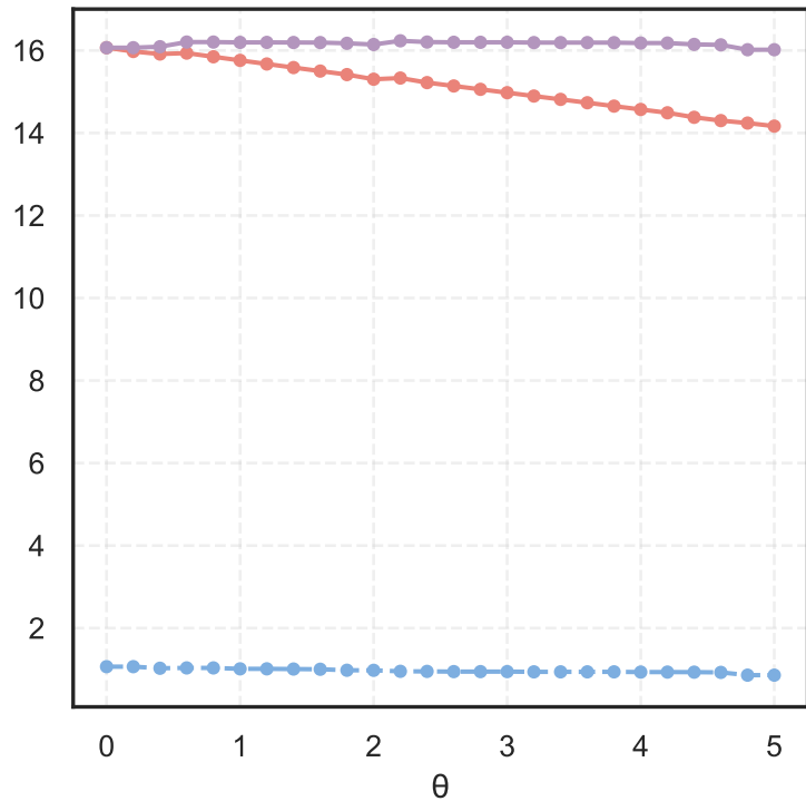
ECC-P
