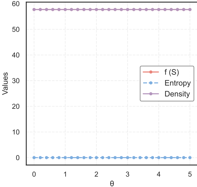
ECC-N
