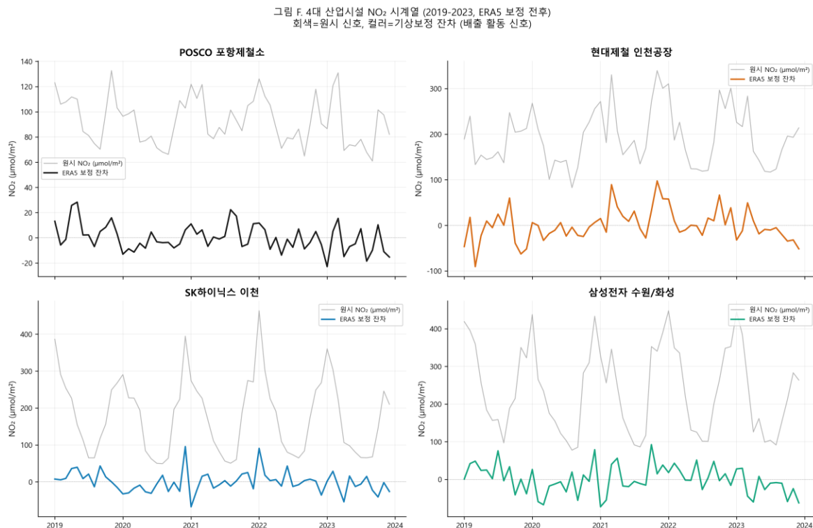
그림 6. 산업시설 네 곳의 NO 2 시계열을 기상보정 전과 후로 비교한 그림입니다. 보정 후에는 계절 진폭이 제거되어 장기 추세가 드러납니다. 중요한 것은 보정 전후 모두에서 핵심 발견의 분류가 변하지 않았다는 점입니다. 즉 이 결과는 보정 방법이 만들어낸 것이 아닙니다.
