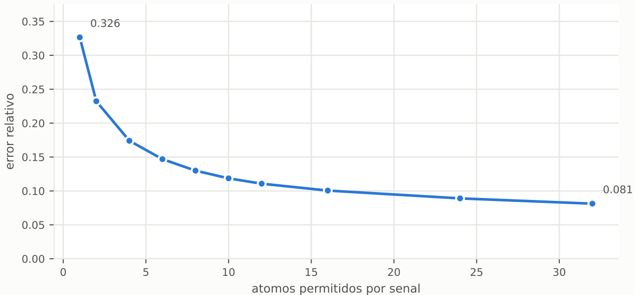
Error de reconstrucción segun el tope de atomos
