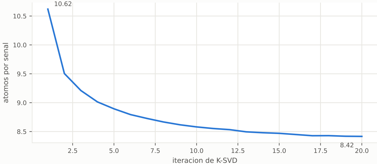
Átomos por señal a lo largo del entrenamiento
