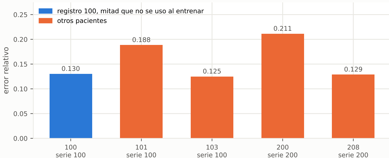
Error con 8 atomos, diccionario entrenado solo con el registro 100
