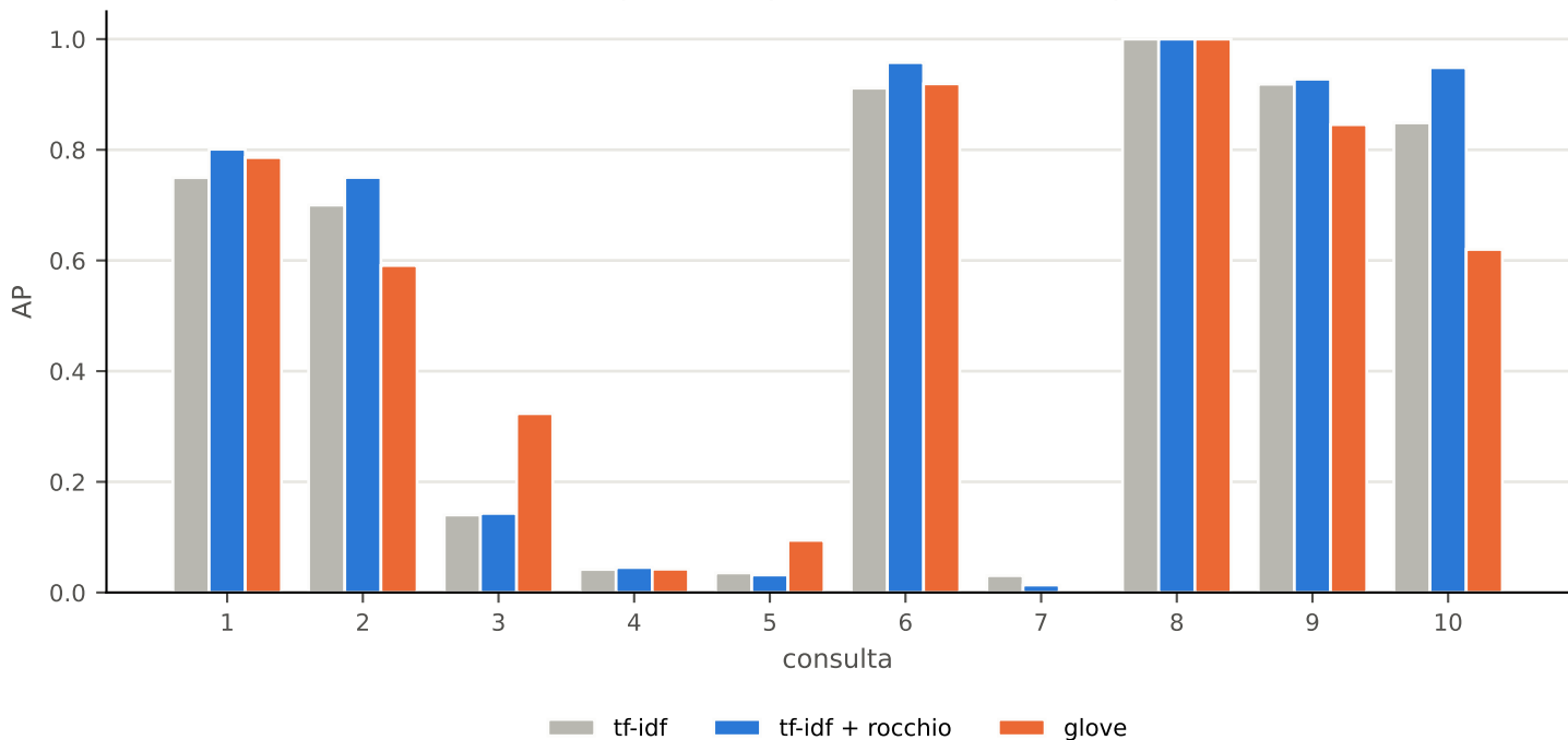
Precision promedio por consulta sobre el top 100
