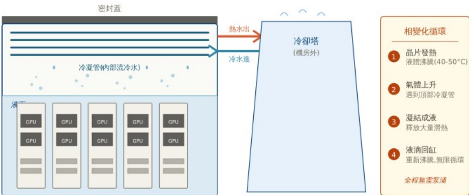
兩相浸沒式冷卻
