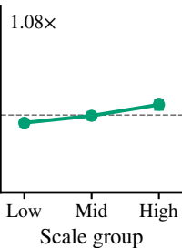
\pi_{0.5} LIBERO
