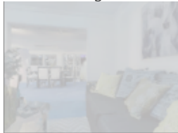
fog
