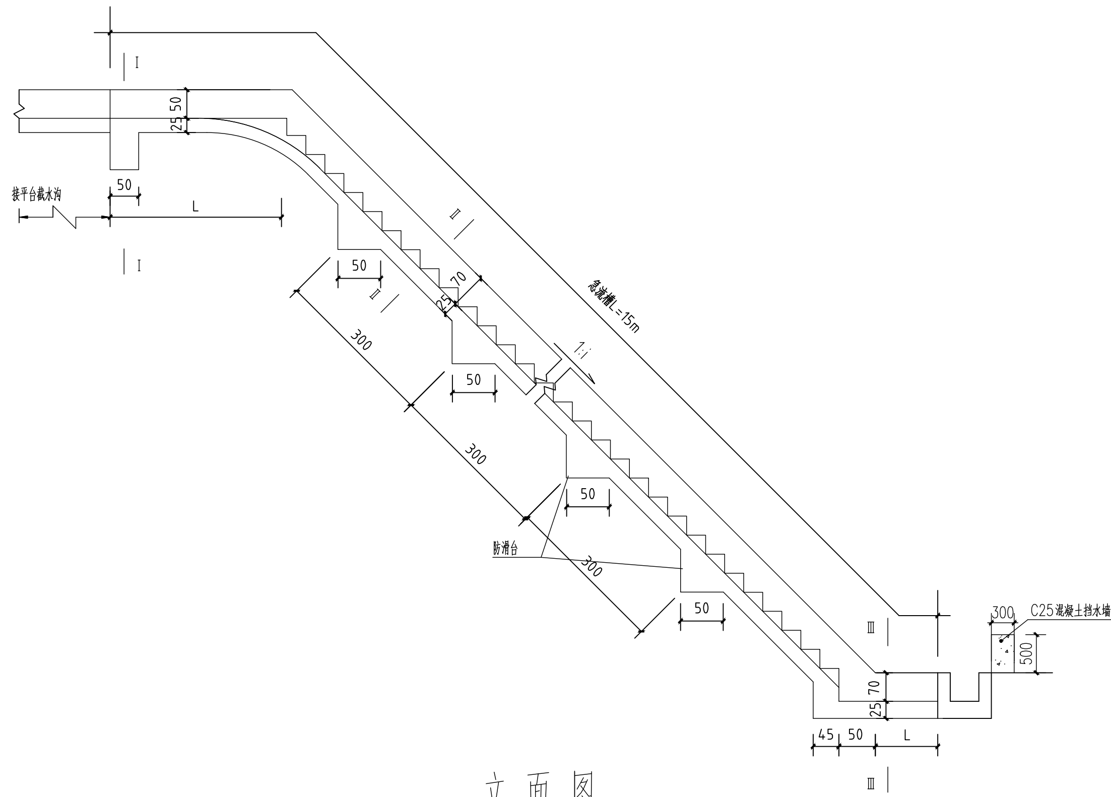
立面图
