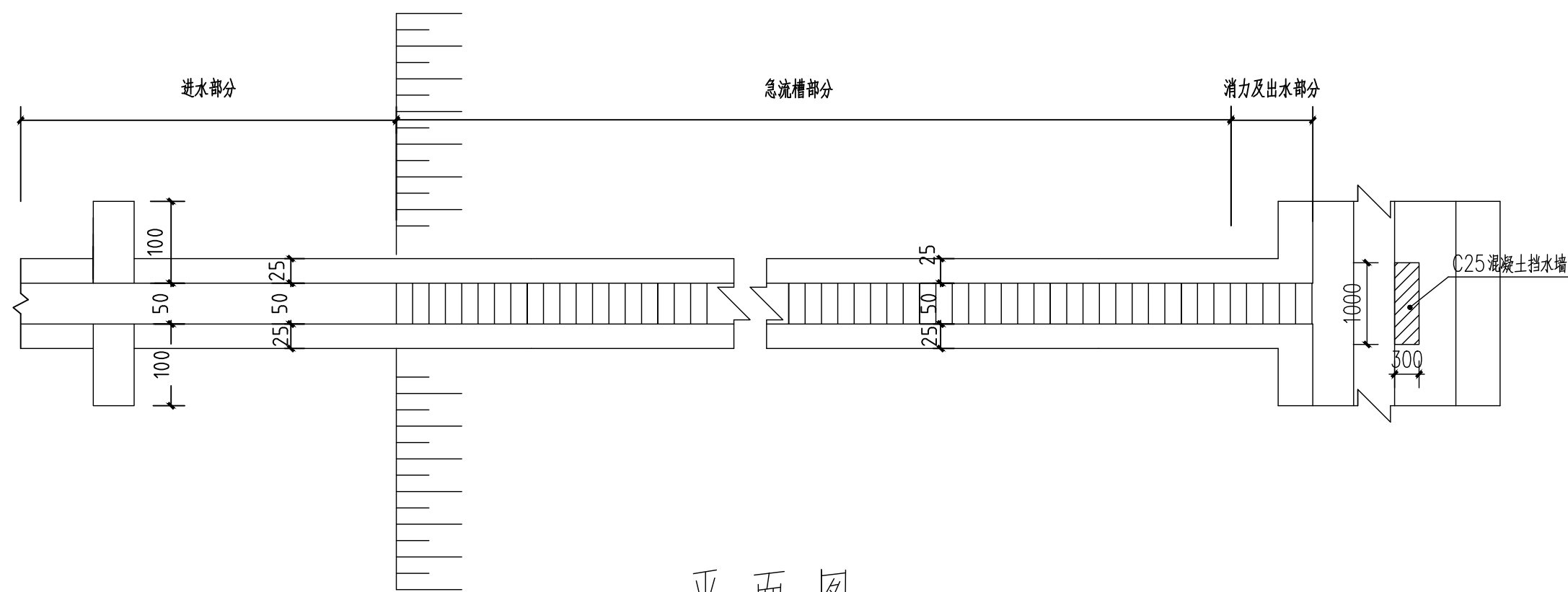
平面图
