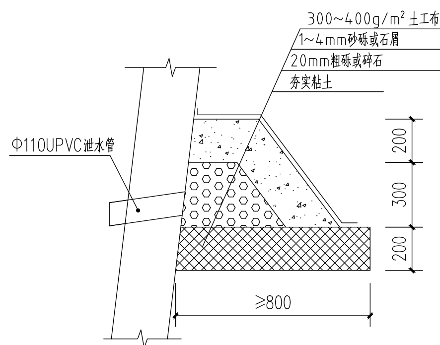
反滤包大样
