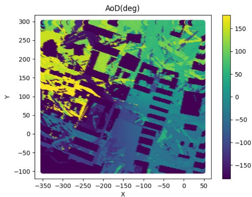
AoD map
