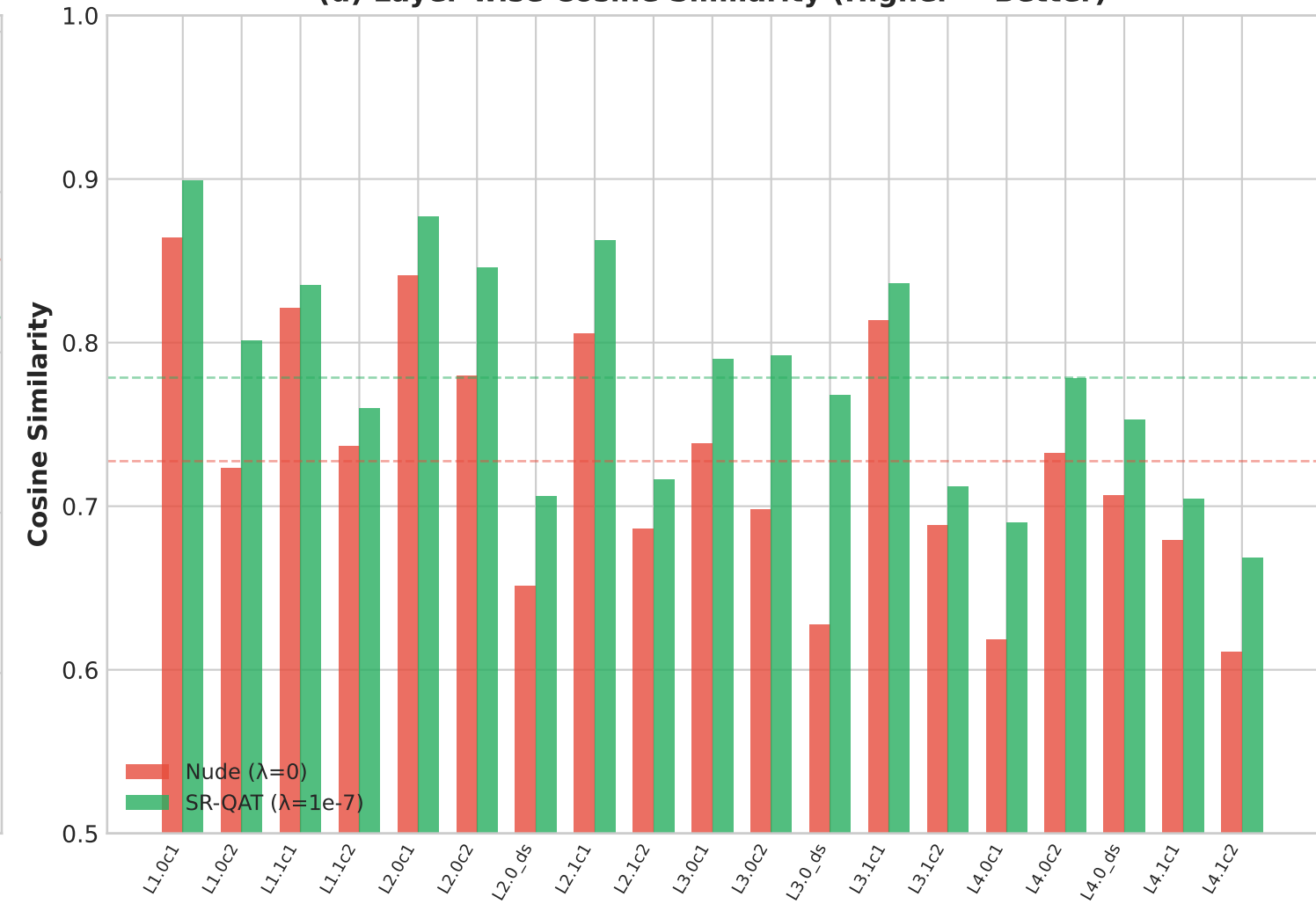
(d) Layer-wise Cosine Similarity (Higher = Better)
