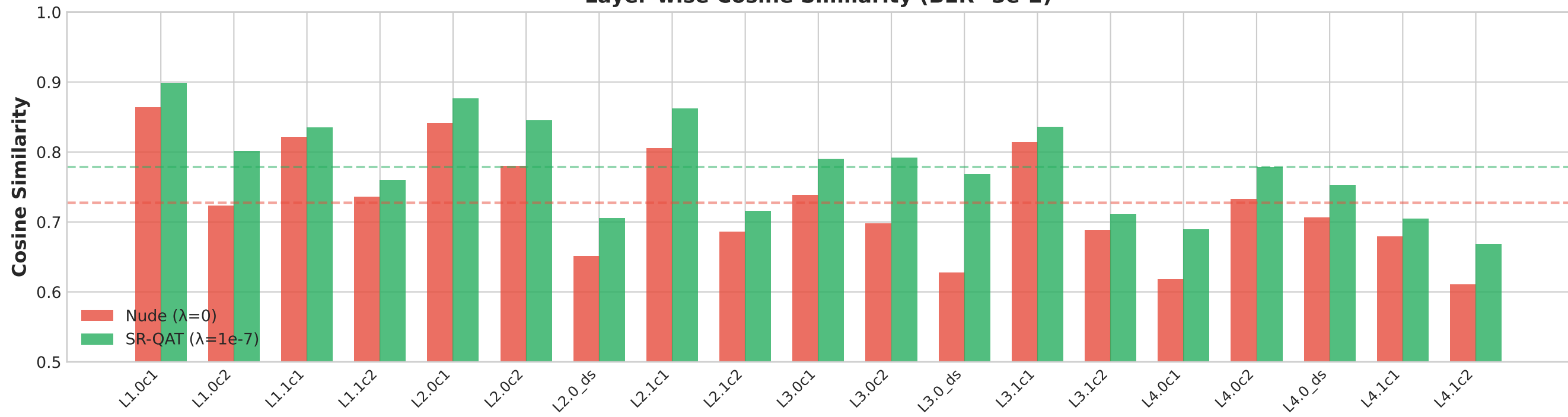
Layer-wise Cosine Similarity (BER=3e-2)
