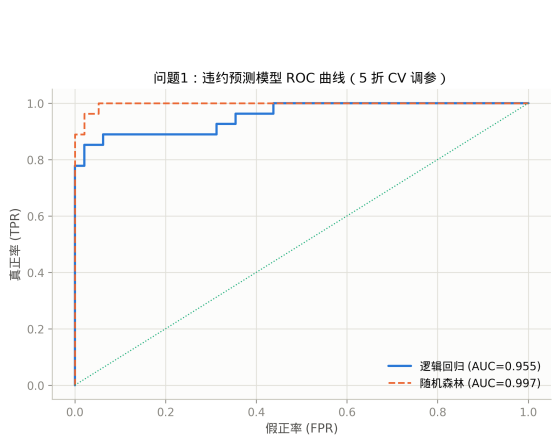
图 4：ROC 曲线
