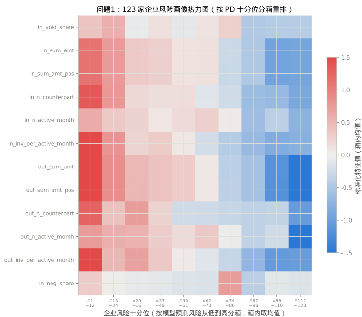
图 6: 123 家企业风险画像热力图 (按 PD 十分位分箱、箱内取均值, 信用风险可视化惯例 [3])
