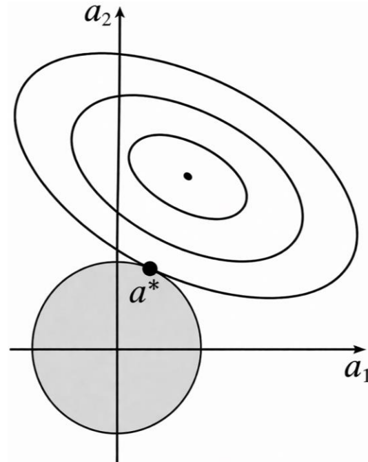
Penalização: norma L2
