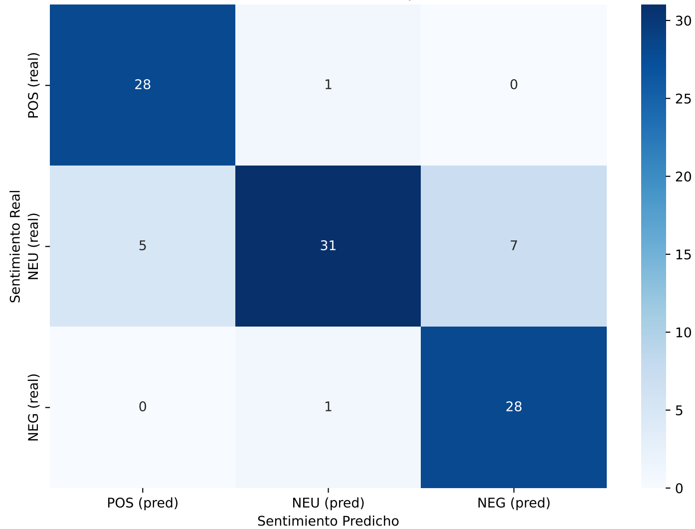
Matriz de Confusión - Accuracy: 86.14%
