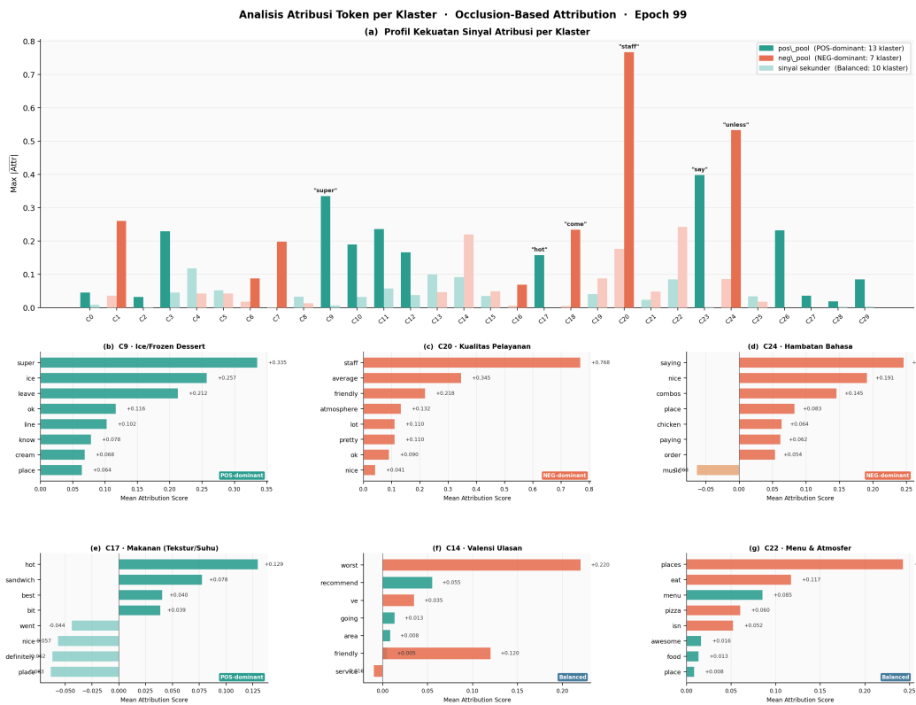
Gambar 4.4: Ringkasan hasil atribusi token pada 30 kluster. Panel (a) menunjukkan nilai atribusi tertinggi pada setiap kluster, sedangkan panel (b)–(g) menampilkan token dengan kontribusi terbesar pada beberapa kluster terpilih berdasarkan skor atribusi rata-rata.
