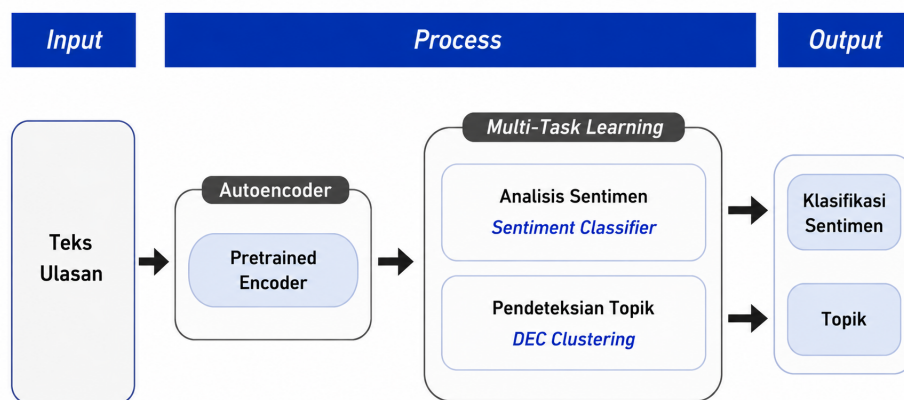
Gambar 3.1: Alur metode analisis sentimen dan pendeteksian topik
