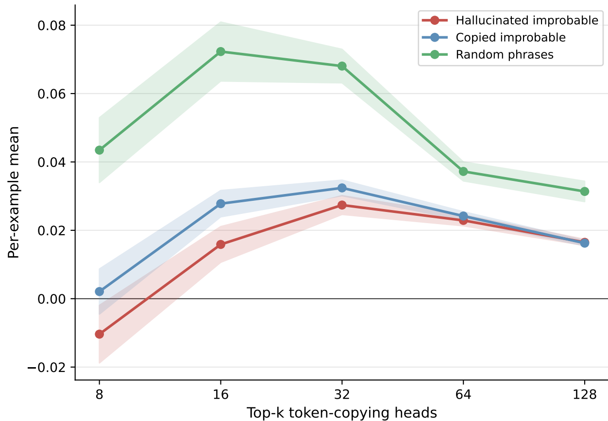
Token correct-token DLA
