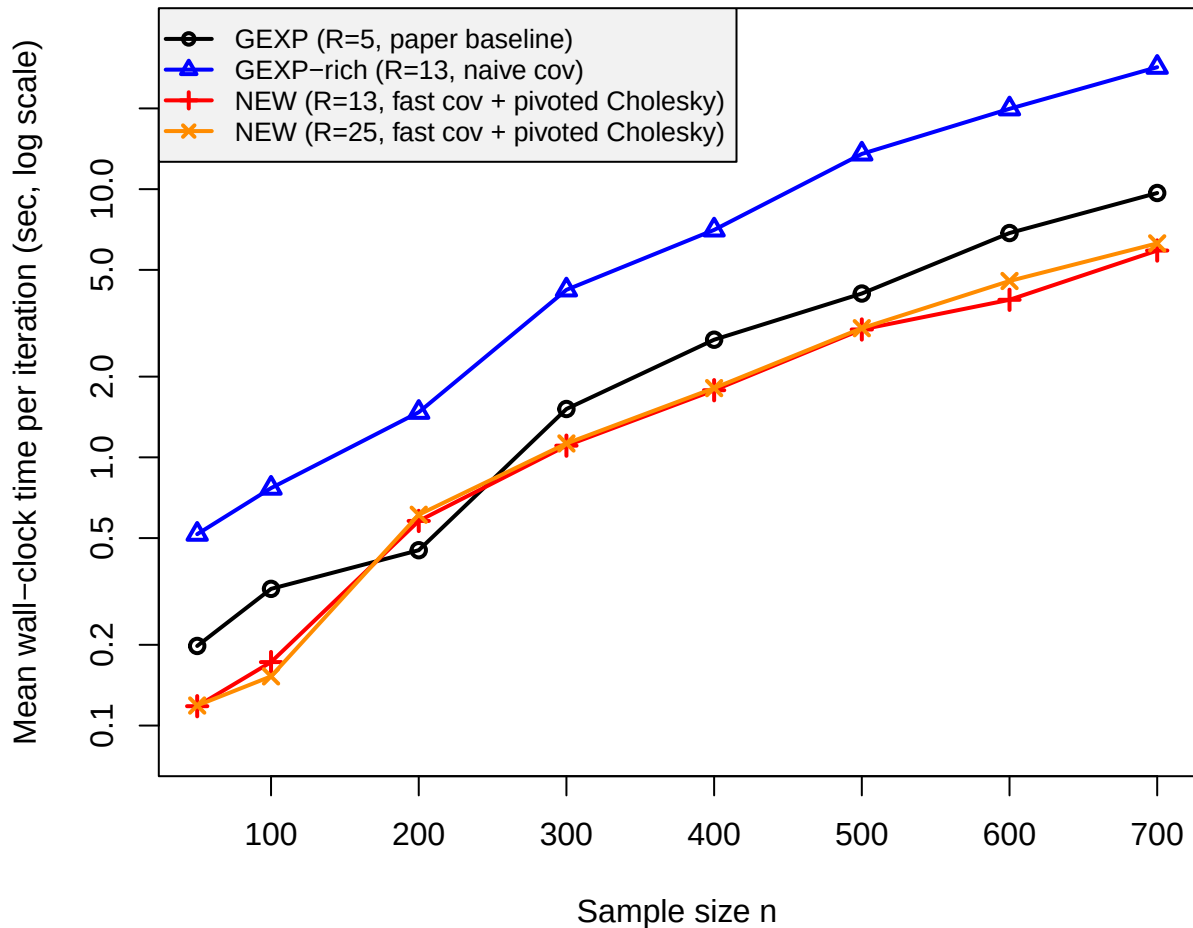
End-to-end time per MC iteration (d = 5, n.iter = 200)
