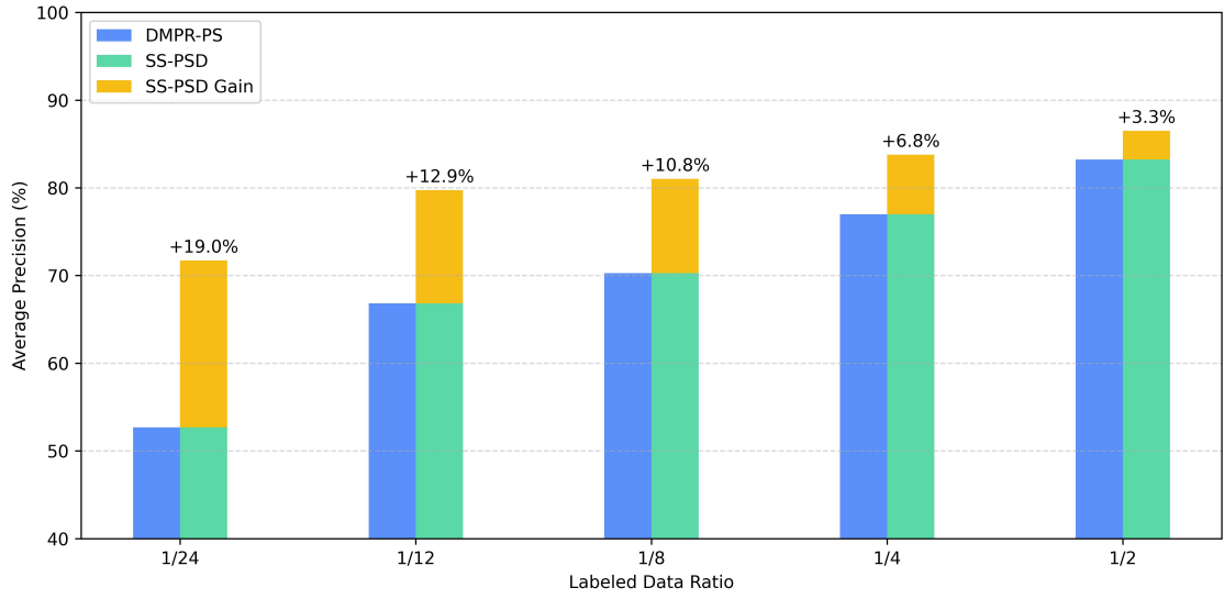
图 3.6 SS-PSD 与 DMPR-PS 的性能比较 (CPRS-D 数据集)
