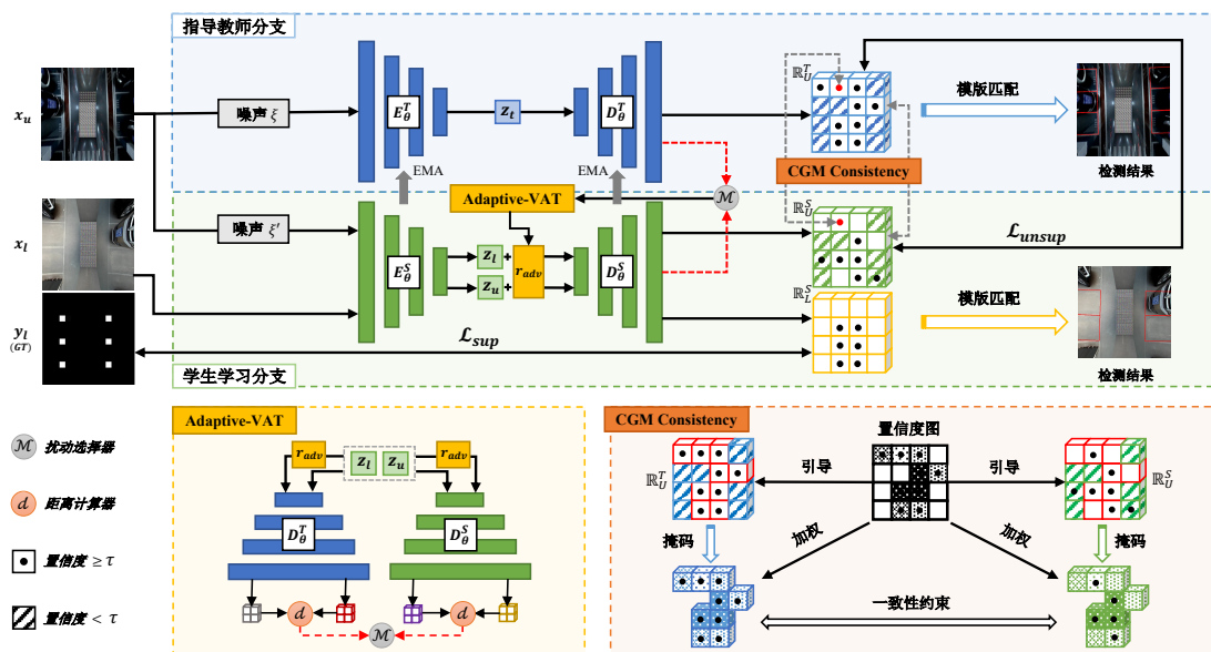
图 3.3 SS-PSD 的整体架构
