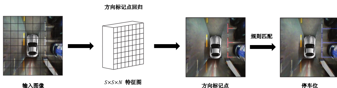
图 1-2 DMPS-PS [14] 算法流程图
