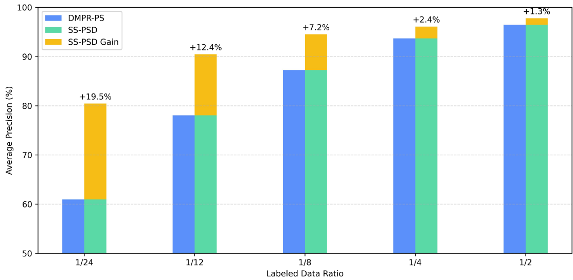
图 3-7 ps2.0 数据集上 SS-PSD 与 DMPR-PS [14] 的性能对比
