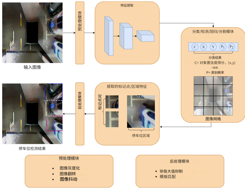
图 2.2 停车位检测的一般流程 [33]
