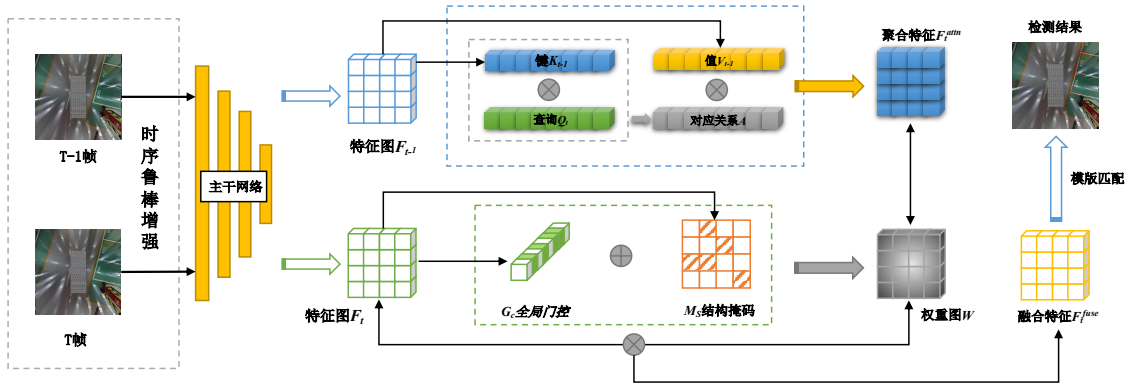
图 5.1 多帧时序特征融合的停车位检测框架示意图
