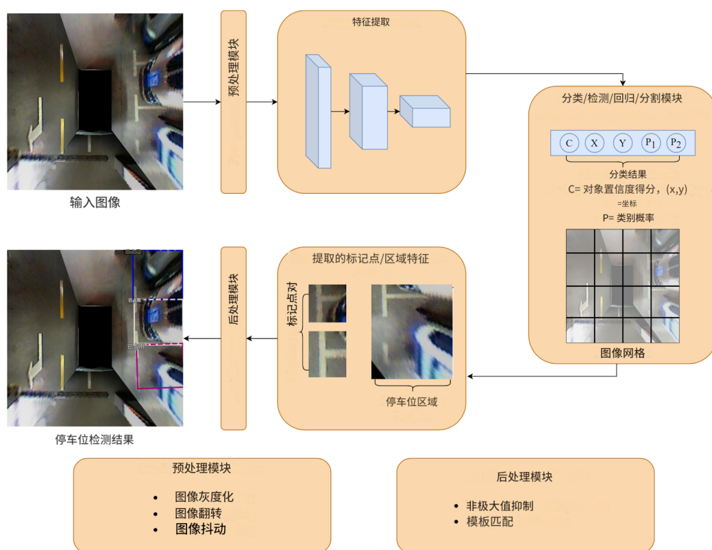
图 2-1 停车位检测的通用框架 [32]
