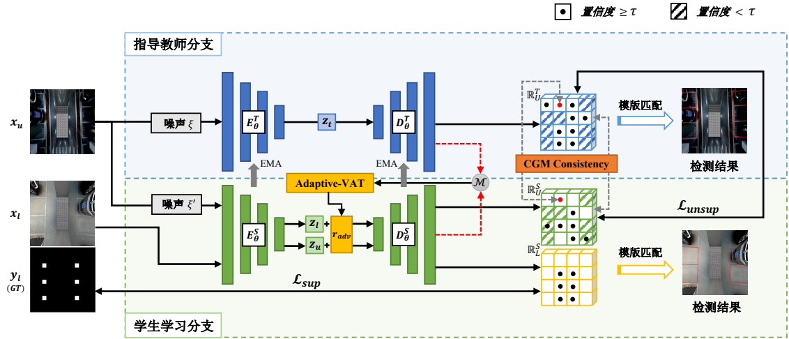
图 3-3 SS-PSD 的整体架构
