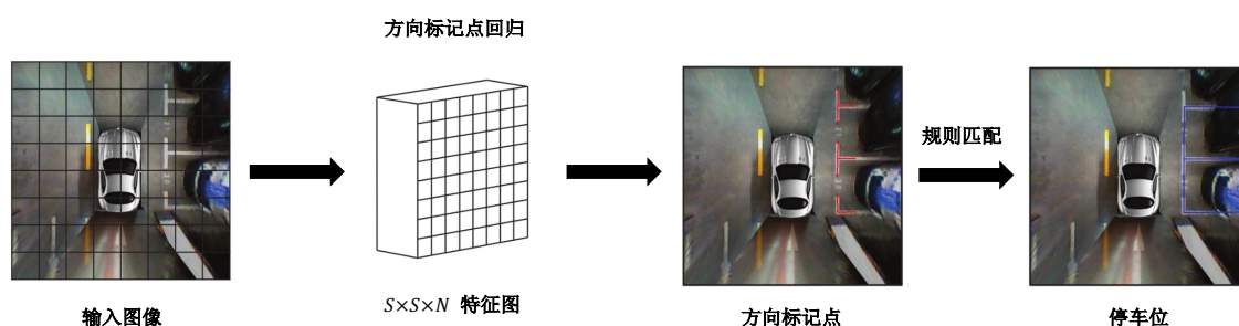
图 1-2 DMPR-PS 算法流程图 [14]
