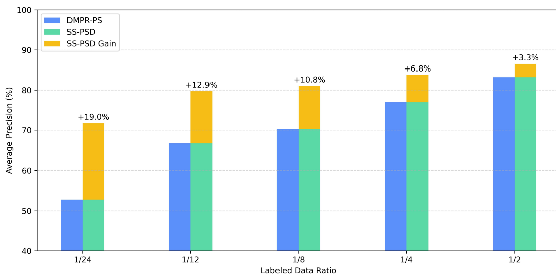
图 3-8 SS-PSD 与 DMPR-PS 的性能比较 (CPRS-D 数据集)
