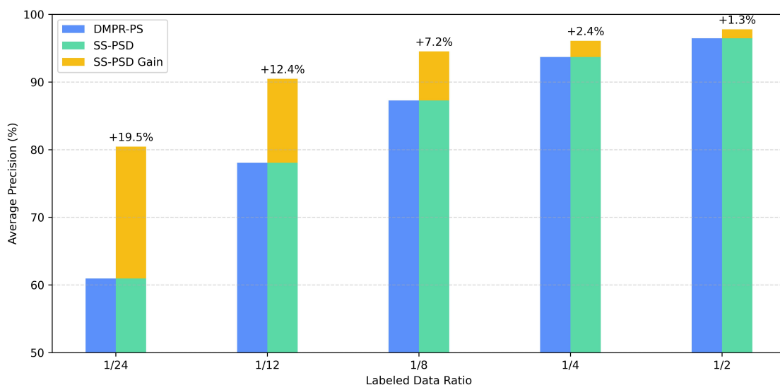
图 3-7 SS-PSD 与 DMPR-PS 的性能比较 (ps2.0 数据集)
