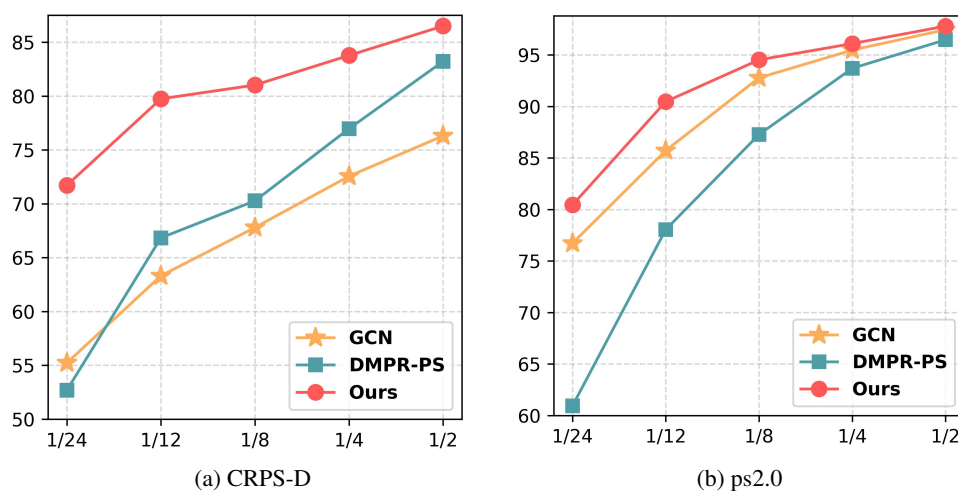
图 3-6 与监督基线相比的改进情况
