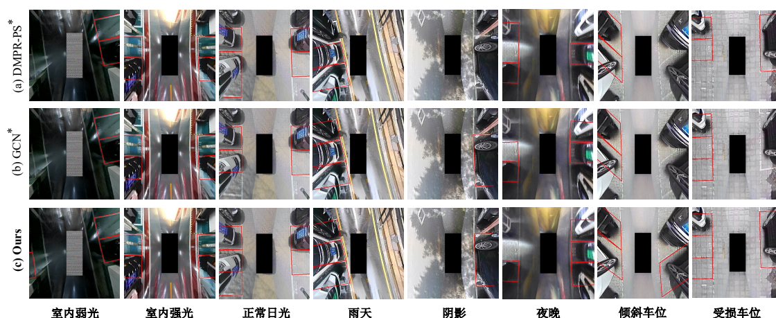
图 3-9 不同场景的可视化结果
