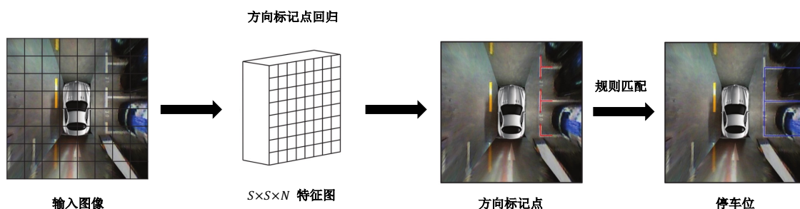
图 1-2 DMPSR-PS [18] 算法流程图
