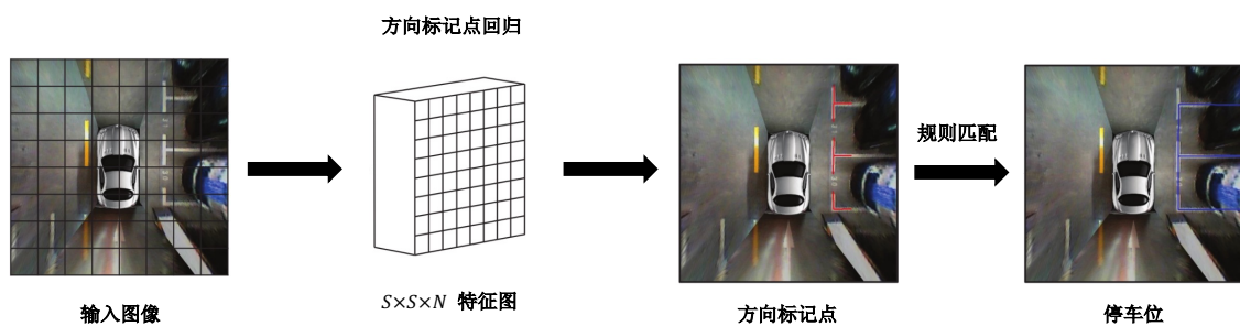
图 1-2 DMPPR-PS [18] 算法流程图
